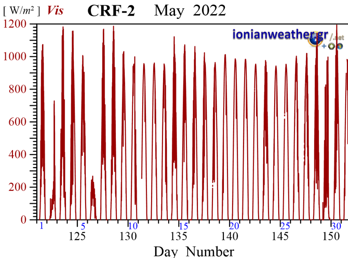
Εικόνα CRF2-7: Μέση ανά λεπτό Ηλιακή ακτινοβολία Μαΐου 2022 στην οπτική περιοχή.
