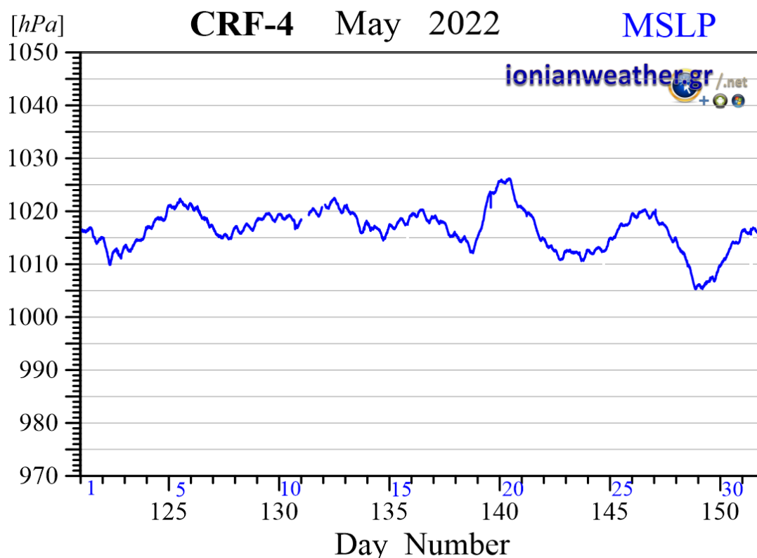
Εικόνα CRF4-6: Μέση ανά λεπτό βαρομετρική πίεση Μαΐου 2022 ανηγμένη στην επιφάνεια της θάλασσας.
