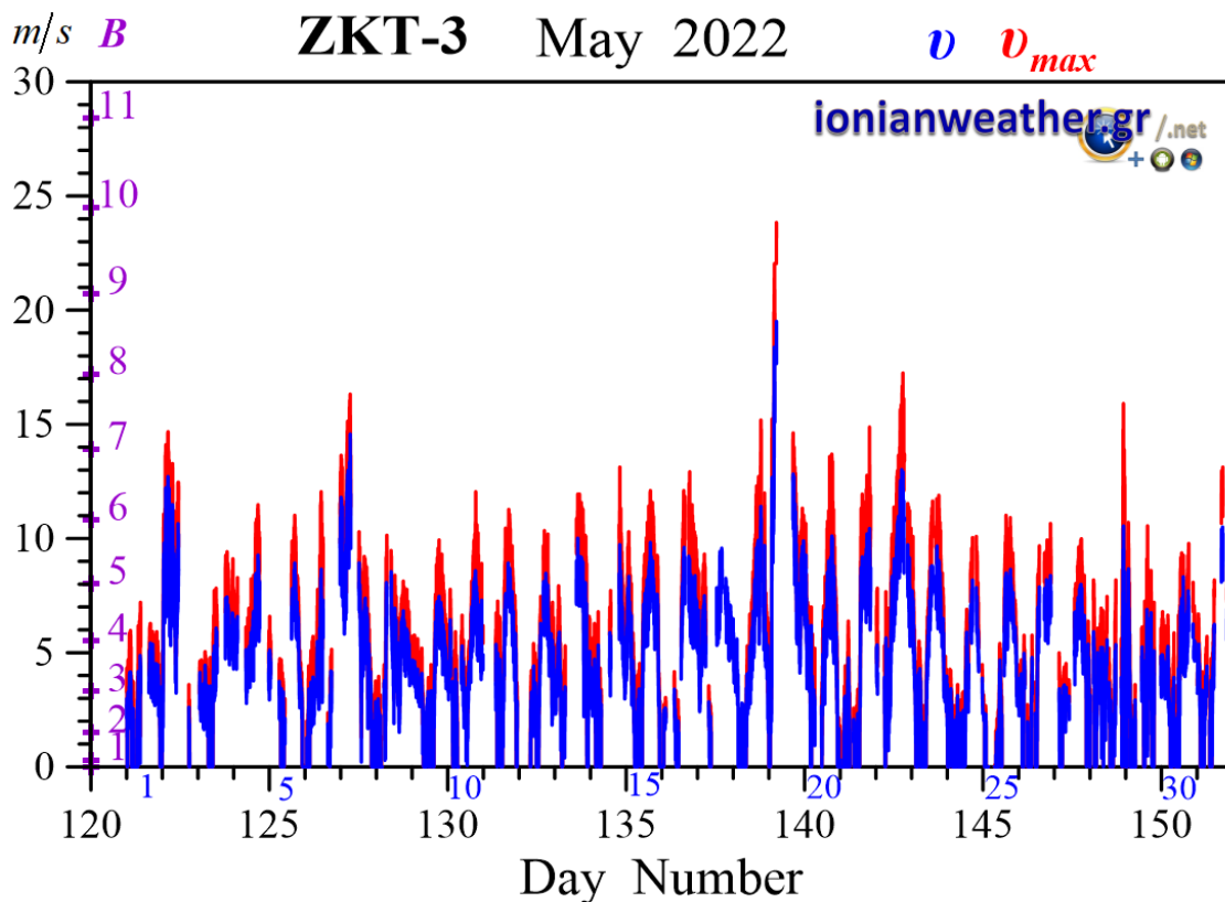
Εικόνα ZKT3-2: Μέση ανά λεπτό ταχύτητα ανέμου ( m/s , γαλάζιο) και ριπή ανέμου (κόκκινο) Μαΐου 2022. Κλίμακα ταχυτήτων αριστερά σε m/s και Beaufort.
