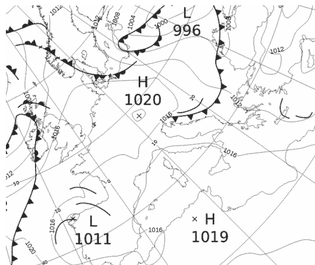
Εικόνα 3.1-22: MSLP 22 May 2022 00UTC
