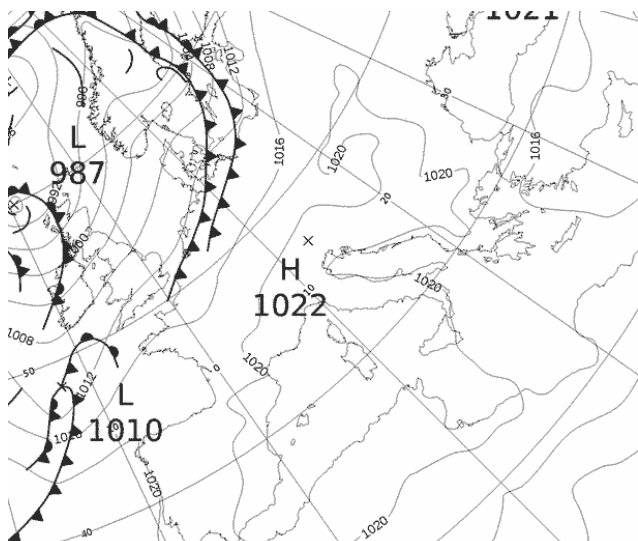
Εικόνα 3.1-11: MSLP 11 May 2022 00UTC
