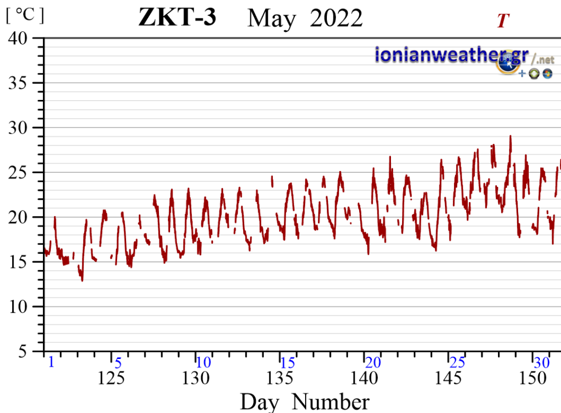
Εικόνα ZKT3-4: Μέση ανά λεπτό θερμοκρασία αέρα Μαΐου 2022.
