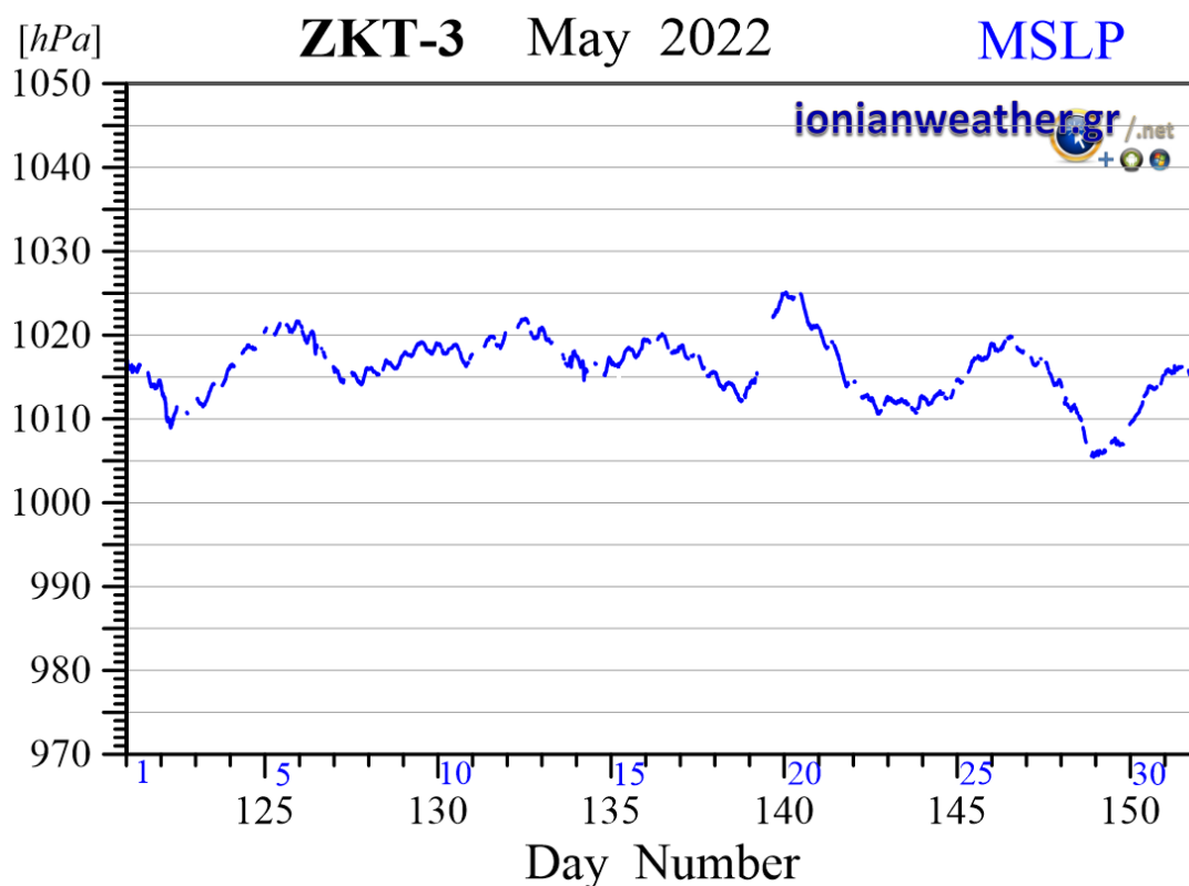
Εικόνα ZKT3-6: Μέση ανά λεπτό βαρομετρική πίεση Μαΐου 2022 ανηγμένη στην επιφάνεια της θάλασσας.
