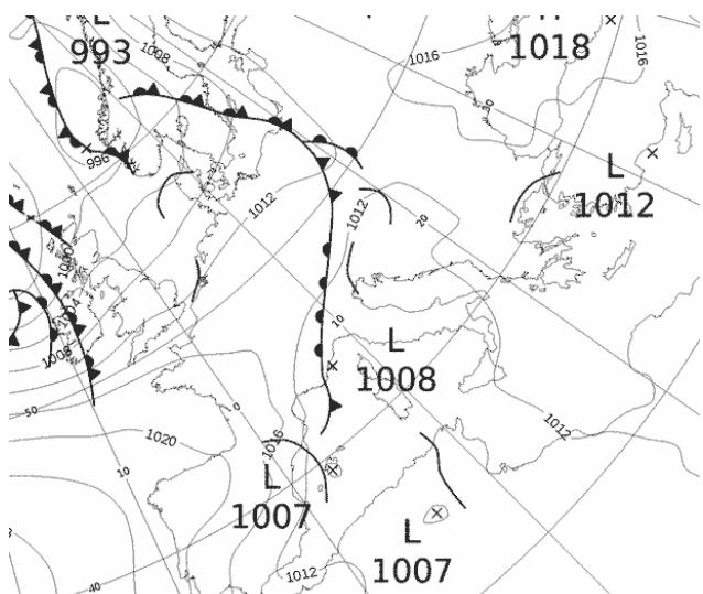
Εικόνα 3.1-25: MSLP 25 May 2022 00UTC
