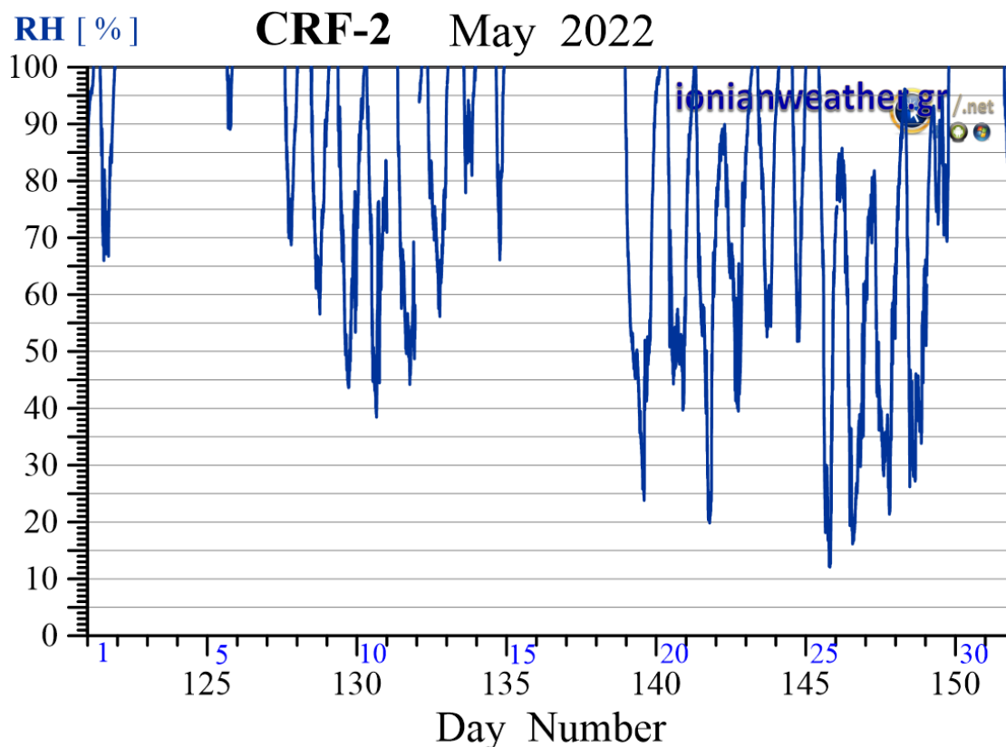
Εικόνα CRF2-5: Μέση ανά λεπτό σχετική υγρασία Μαΐου 2022.
