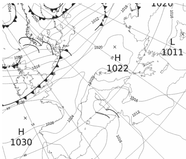
Εικόνα 3.1-27: MSLP 27 May 2022 00UTC
