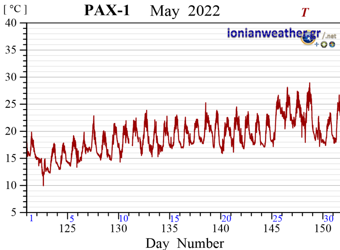
Εικόνα PAX 1-4: Μέση ανά λεπτό θερμοκρασία αέρα Μαΐου 2022.
