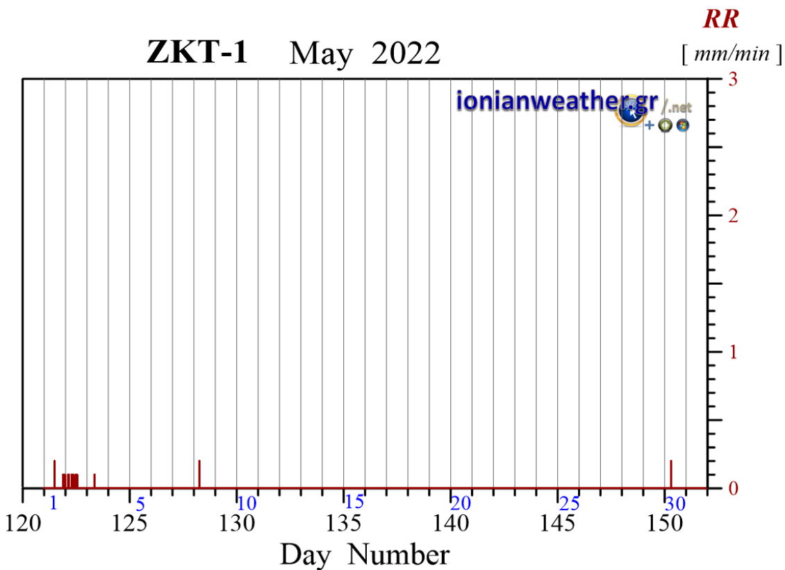
Εικόνα ZKT1-1: Ανά λεπτό ρυθμός βροχόπτωσης (mm/min) Μαΐου 2022.
