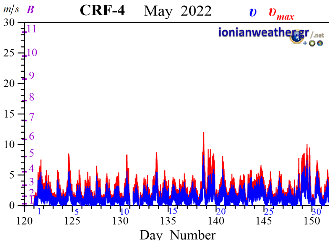
Εικόνα CRF4-2: Μέση ανά λεπτό ταχύτητα ανέμου ( m/s , γαλάζιο) και ριπή ανέμου (κόκκινο) Μαΐου 2022. Κλίμακα ταχυτήτων αριστερά σε m/s και Beaufort .
