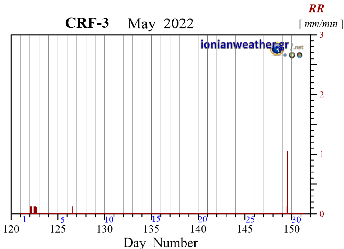
Εικόνα CRF3-1: Ανά λεπτό ρυθμός βροχόπτωσης (mm/min) Μαΐου 2022.
