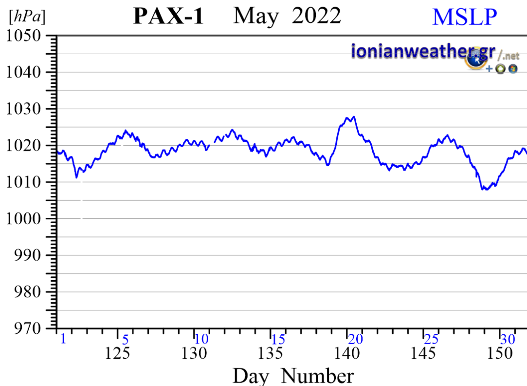
Εικόνα PAX 1-5: Μέση ανά λεπτό βαρομετρική πίεση Μαΐου 2022 ανηγμένη στην επιφάνεια της θάλασσας.
