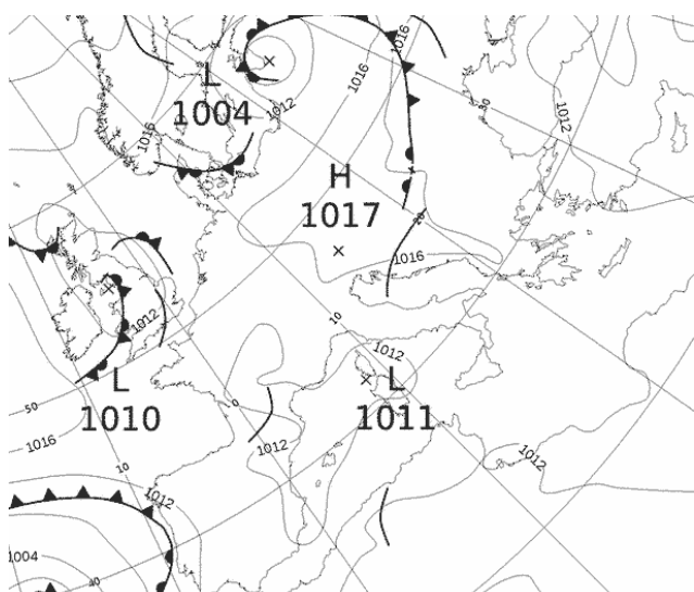
Εικόνα 3.1-31: MSLP 31 May 2022 00UTC
