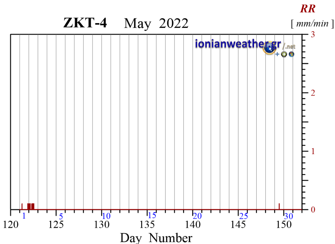
Εικόνα ZKT4-1: Ανά λεπτό ρυθμός βροχόπτωσης (mm/min) Μαΐου 2022.
