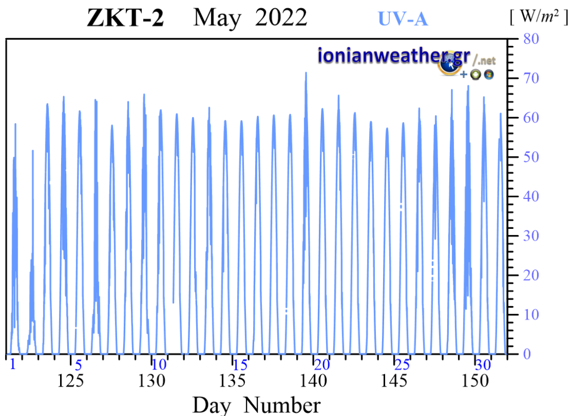
Εικόνα ZKT2-8: Μέση ανά λεπτό Ηλιακή ακτινοβολία Μαΐου 2022 στη φασματική περιοχή UVA.
