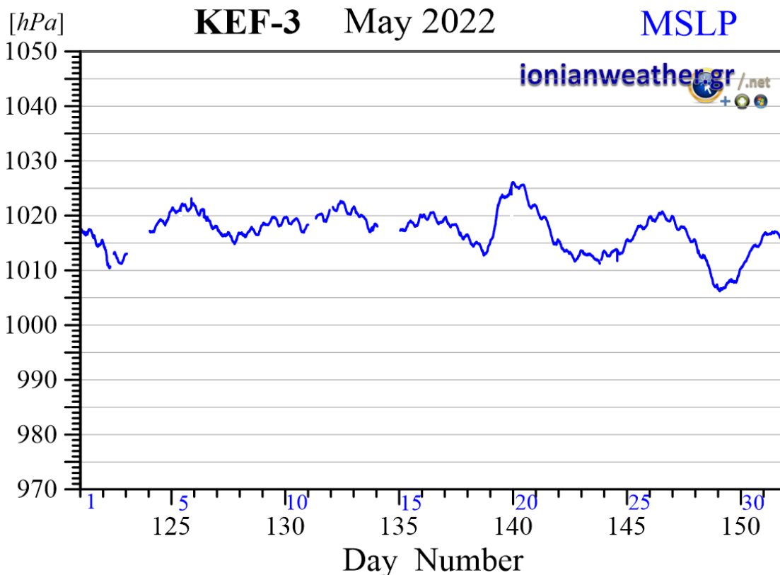
Εικόνα KEF3-6: Μέση ανά λεπτό βαρομετρική πίεση Μαΐου 2022 ανηγμένη στην επιφάνεια της θάλασσας.
