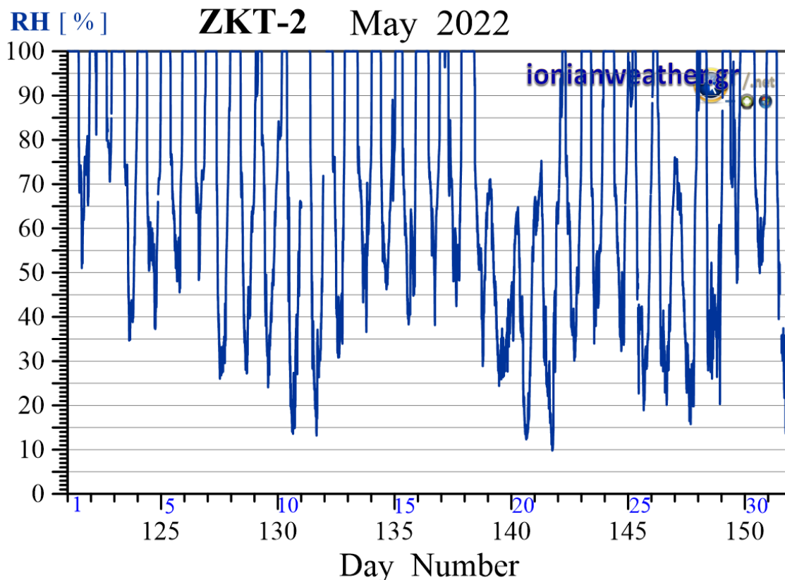
Εικόνα ZKT2-5: Μέση ανά λεπτό σχετική υγρασία Μαΐου 2022.
