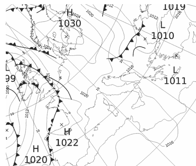
Εικόνα 3.1-18: MSLP 18 May 2022 00UTC
