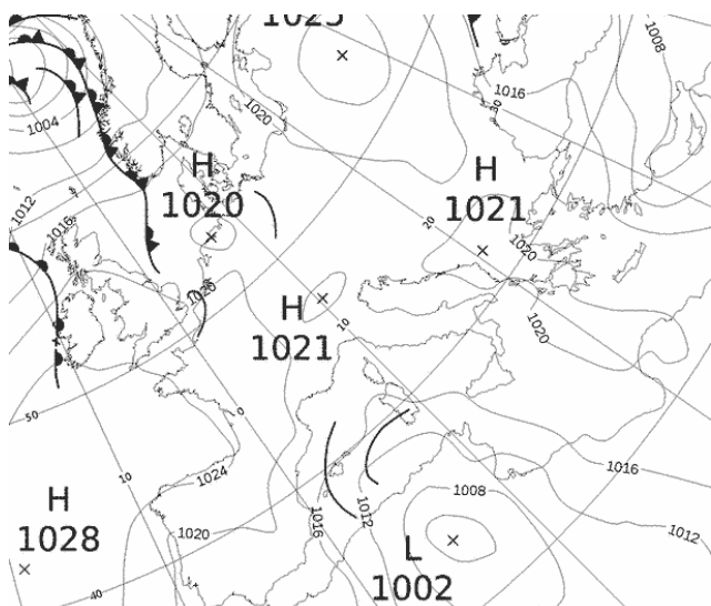
Εικόνα 3.1-5: MSLP 5 May 2022 00UTC
