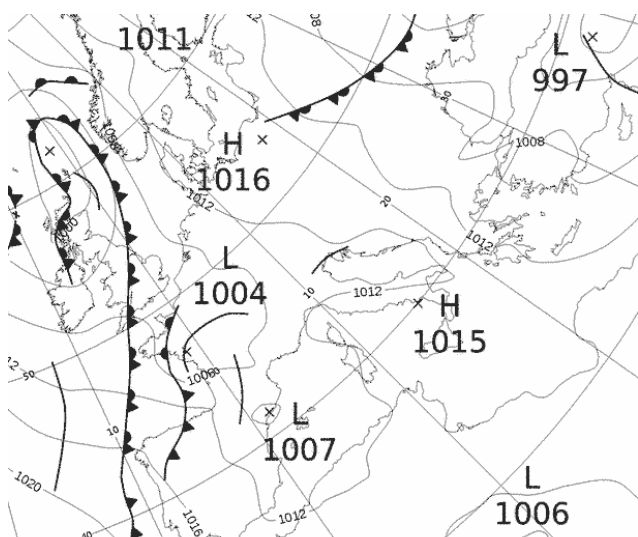
Εικόνα 3.1-23: MSLP 23 May 2022 00UTC
