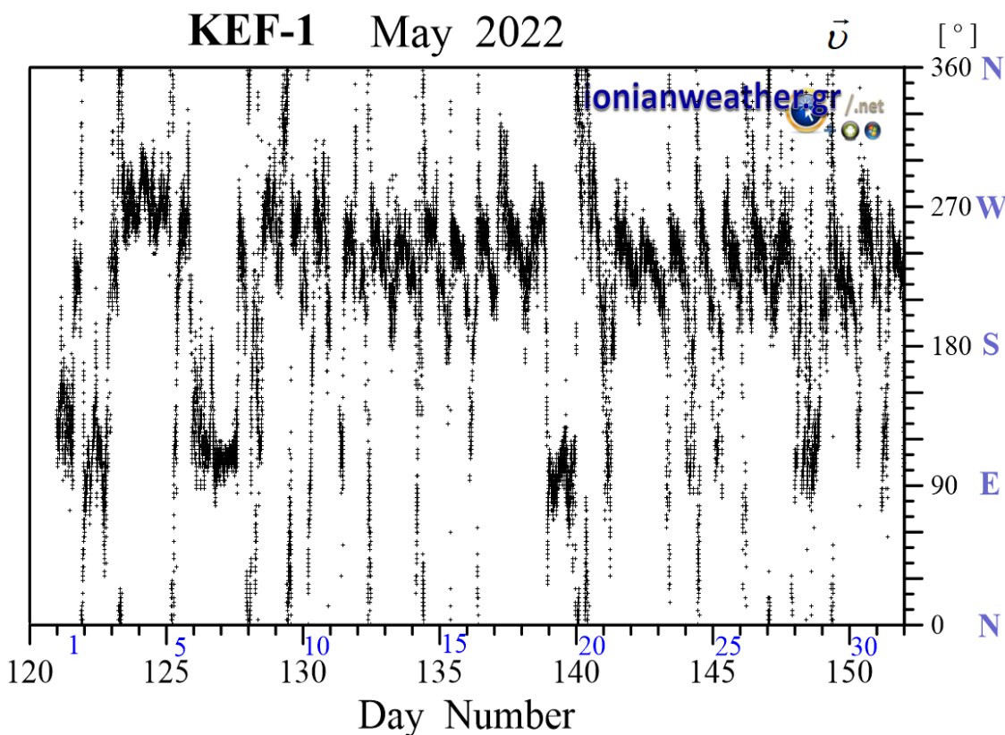
Εικόνα KEF1-3: Μέση ανά λεπτό κατεύθυνση ανέμου Μαΐου 2022 (κλίμακα αζιμουθίων δεξιά)
