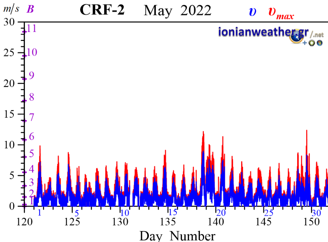
Εικόνα CRF2-2: Μέση ανά λεπτό ταχύτητα ανέμου ( m/s , γαλάζιο) και ριπή ανέμου (κόκκινο) Μαΐου 2022. Κλίμακα ταχυτήτων αριστερά σε m/s και Beaufort.
