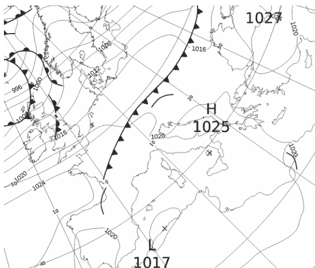
Εικόνα 3.1-13: MSLP 13 May 2022 00UTC
