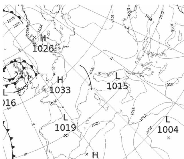
Εικόνα 3.1-1: MSLP 1 May 2022 00UTC
