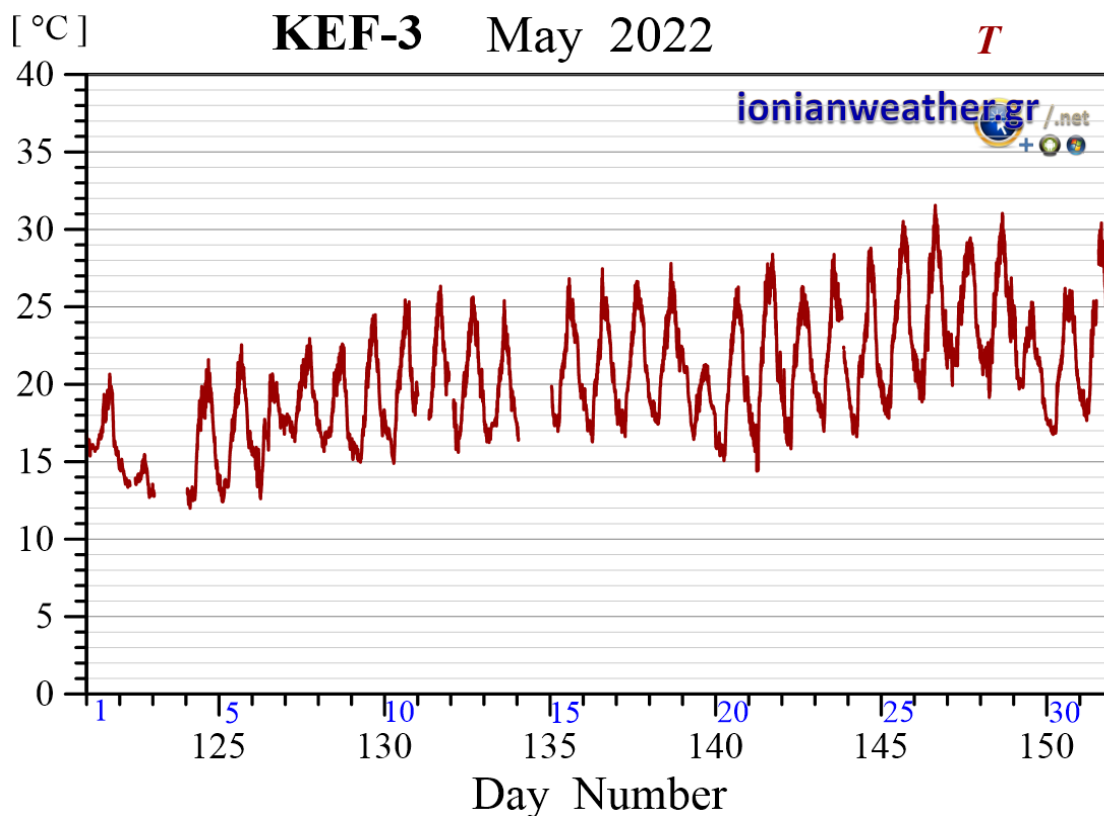
Εικόνα KEF3-4: Μέση ανά λεπτό θερμοκρασία αέρα Μαΐου 2022.
