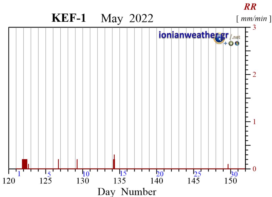
Εικόνα KEF1-1: Ανά λεπτό ρυθμός βροχόπτωσης (mm/min) Μαΐου 2022.
