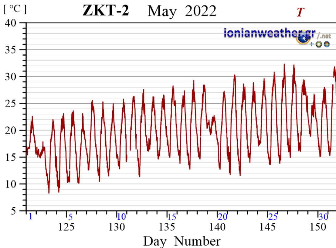
Εικόνα ZKT2-4: Μέση ανά λεπτό θερμοκρασία αέρα Μαΐου 2022.
