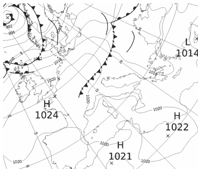
Εικόνα 3.1-14: MSLP 14 May 2022 00UTC
