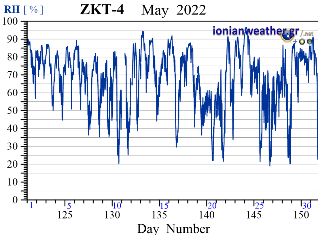
Εικόνα ZKT4-5: Μέση ανά λεπτό σχετική υγρασία Μαΐου 2022.
