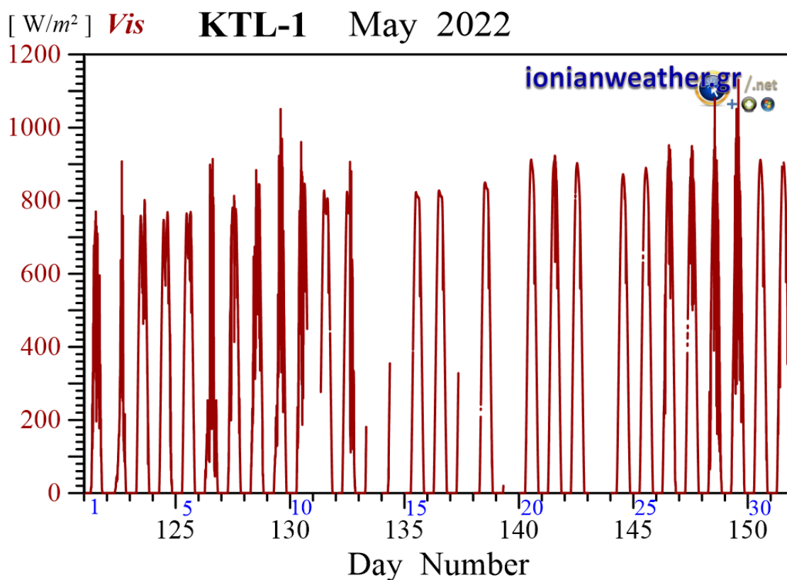
Εικόνα KTL1-7: Μέση ανά λεπτό Ηλιακή ακτινοβολία Μαΐου 2022 στην οπτική και εγγύς υπέρυθρη περιοχή.
