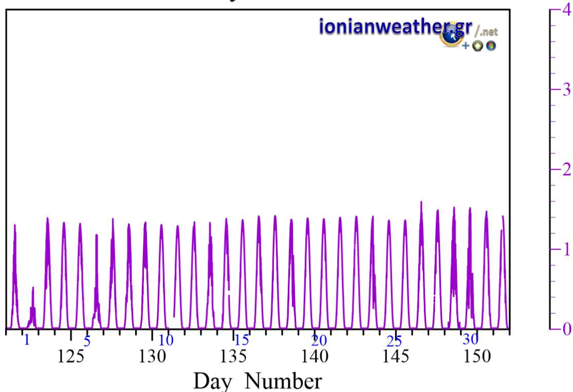
Εικόνα KEF1-9: Μέση ανά λεπτό Ηλιακή ακτινοβολία Μαΐου 2022 στη φασματική περιοχή UVB
