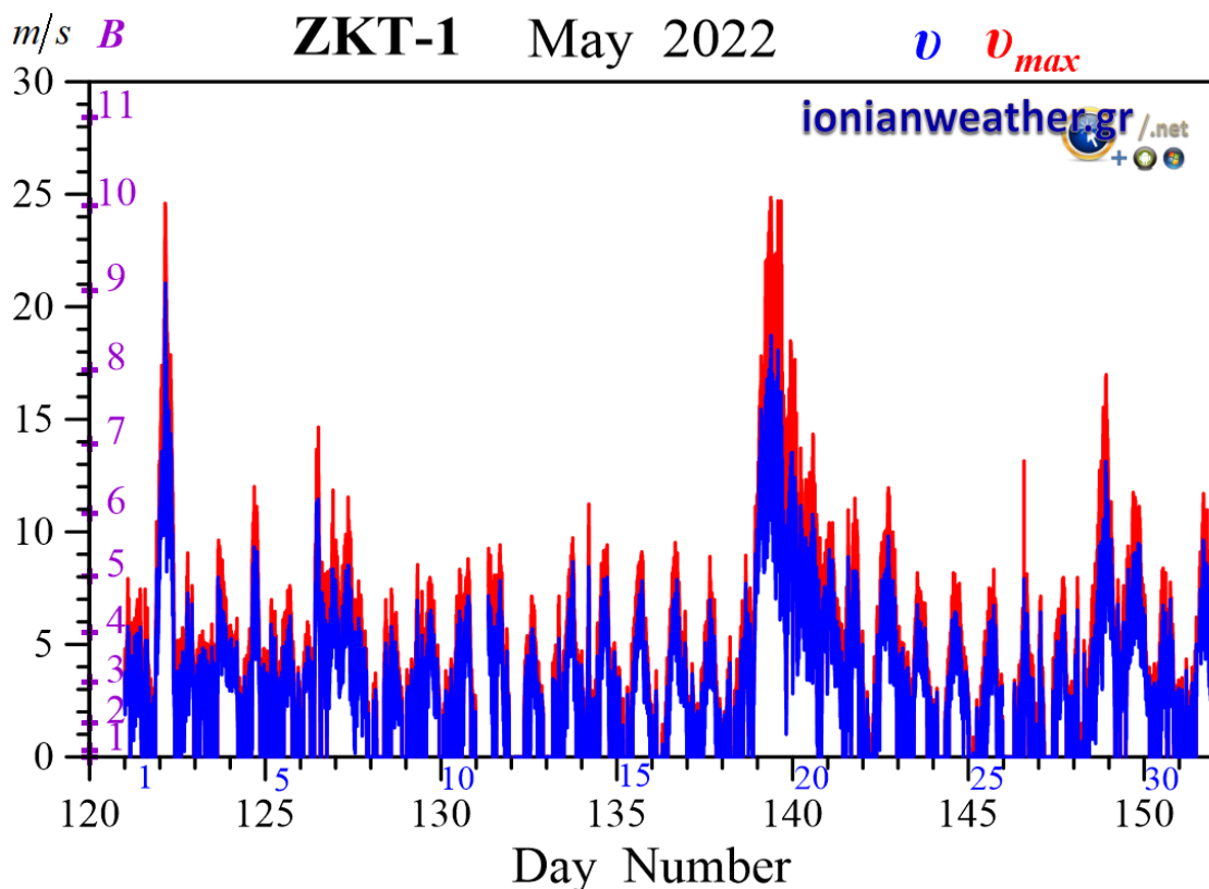
Εικόνα ZKT1-2: Μέση ανά λεπτό ταχύτητα ανέμου ( m/s , γαλάζιο) και ριπή ανέμου (κόκκινο) Μαΐου 2022. Κλίμακα ταχυτήτων αριστερά σε m/s και Beaufort.
