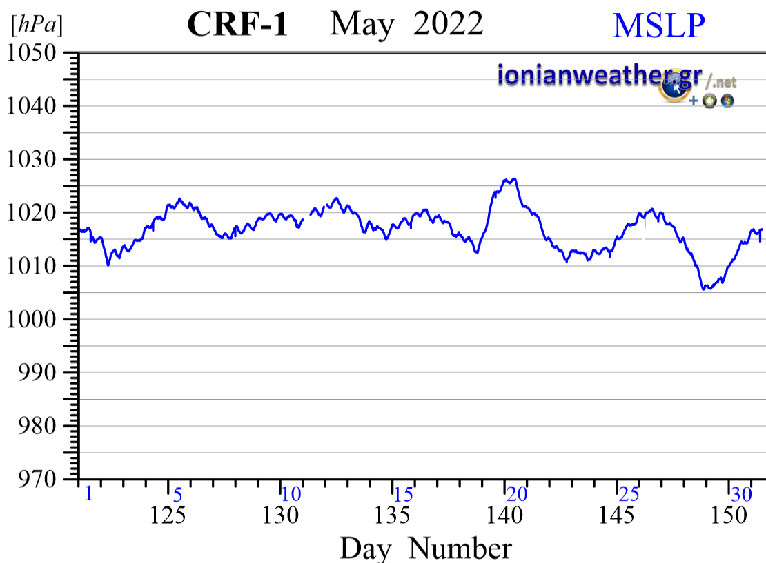
Εικόνα CRF1-6: Μέση ανά λεπτό βαρομετρική πίεση Μαΐου 2022 ανηγμένη στην επιφάνεια της θάλασσας.
