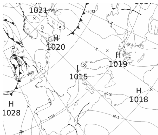
Εικόνα 3.1-4: MSLP 4 May 2022 00UTC
