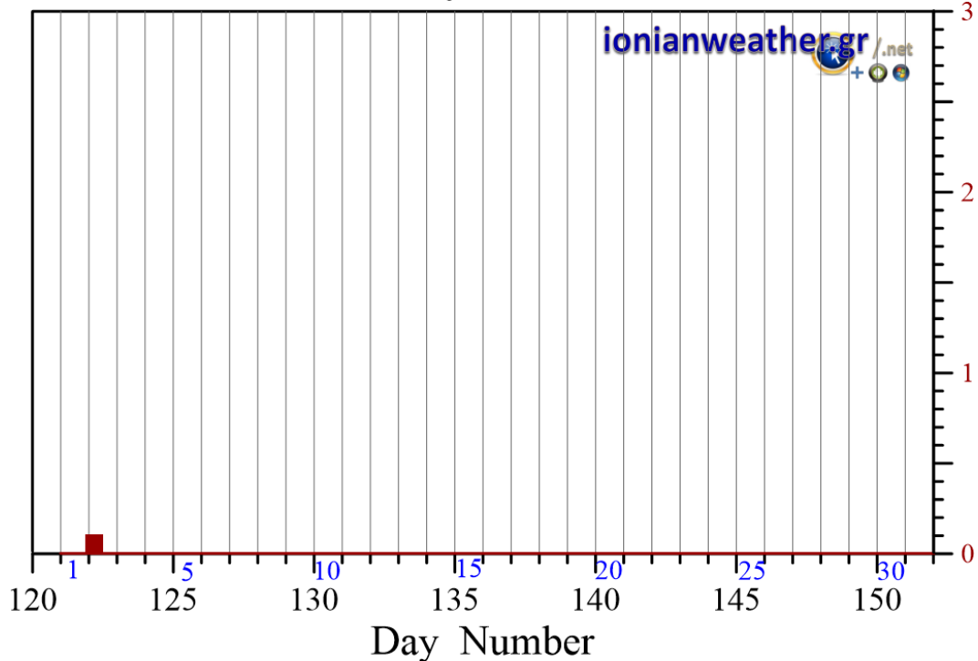
Εικόνα ZKT3-1: Ανά λεπτό ρυθμός βροχόπτωσης (mm/min) Μαΐου 2022.
