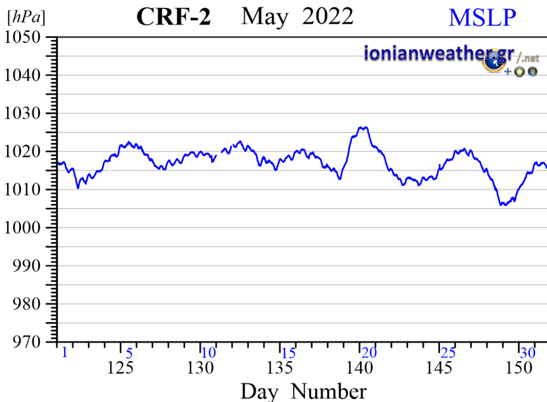
Εικόνα CRF2-6: Μέση ανά λεπτό βαρομετρική πίεση Μαΐου 2022 ανηγμένη στην επιφάνεια της θάλασσας.
