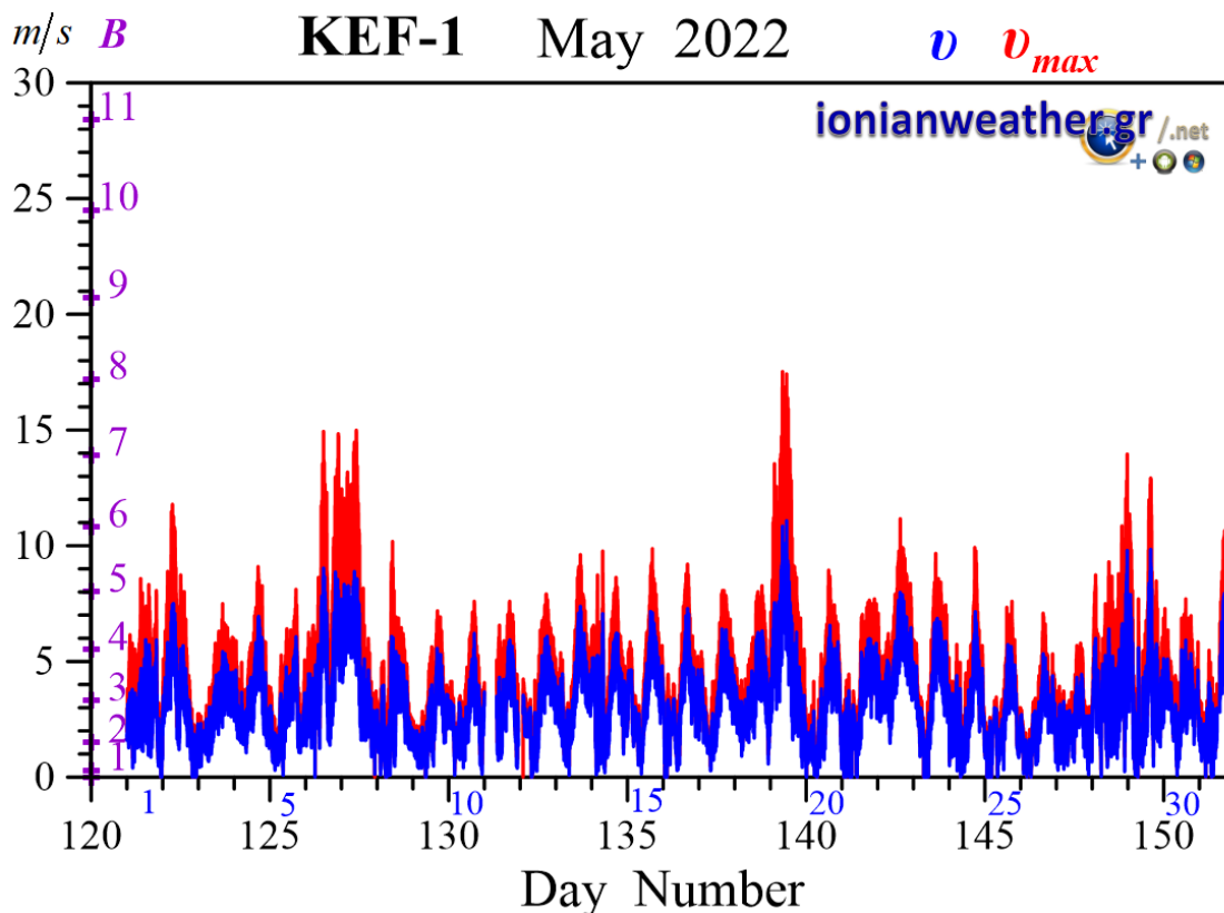
Εικόνα KEF1-2: Μέση ανά λεπτό ταχύτητα ανέμου ( m/s , γαλάζιο) και ριπή ανέμου (κόκκινο) Μαΐου 2022. Κλίμακα ταχυτήτων αριστερά σε m/s και Beaufort.
