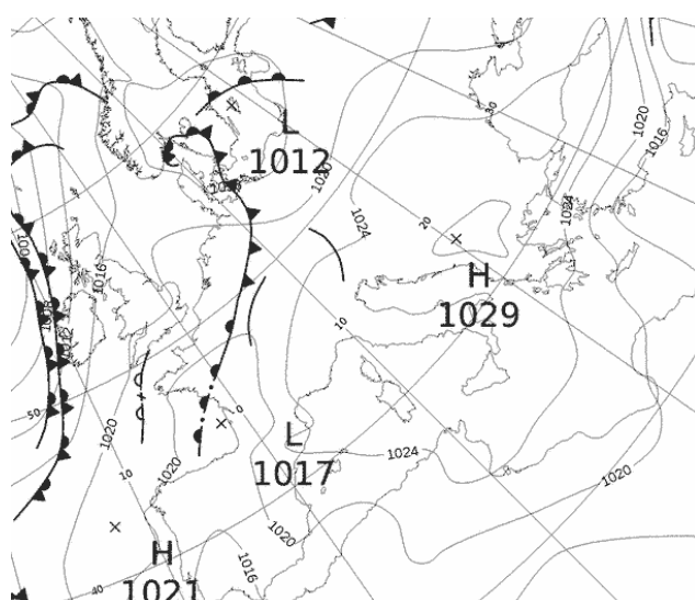
Εικόνα 3.1-20: MSLP 20 May 2022 00UTC
