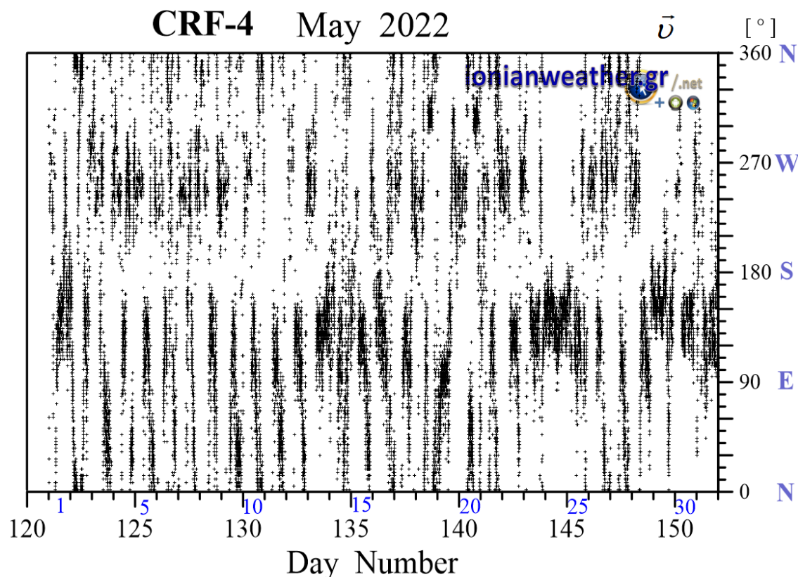
Εικόνα CRF4-3: Μέση ανά λεπτό κατεύθυνση ανέμου Μαΐου 2022 (κλίμακα αζιμουθίων δεξιά)
