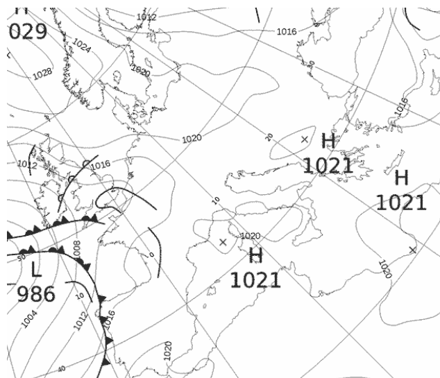
Εικόνα 3.1-16: MSLP 16 May 2022 00UTC
