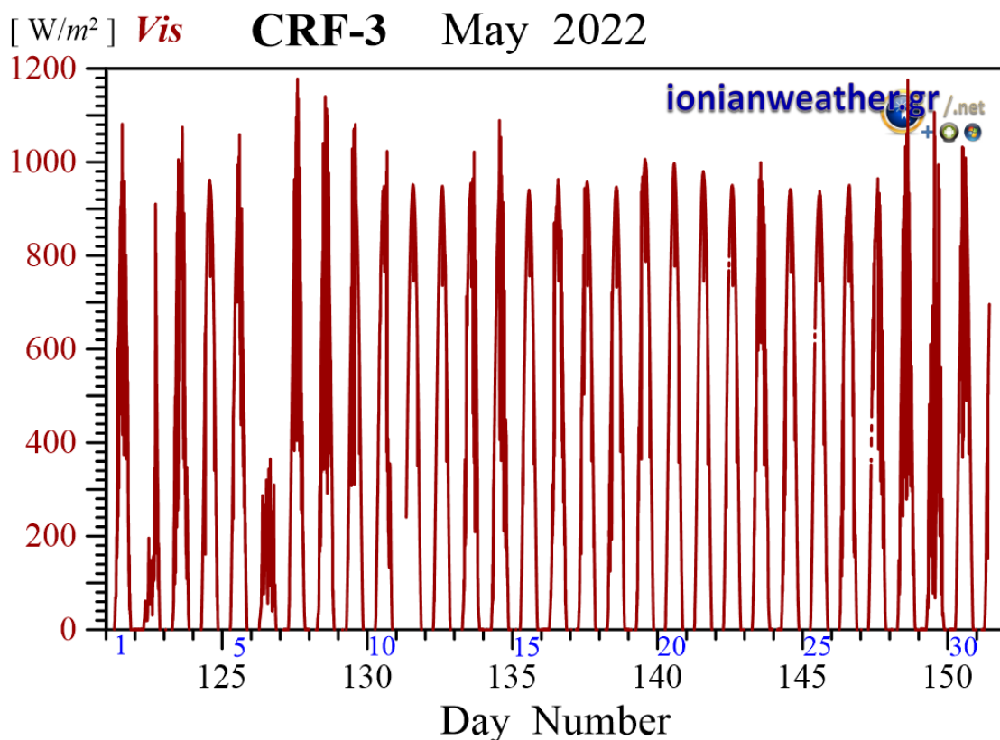
Εικόνα CRF3-7: Μέση ανά λεπτό Ηλιακή ακτινοβολία Μαΐου 2022 στην οπτική και εγγύς υπέρυθρη περιοχή.
