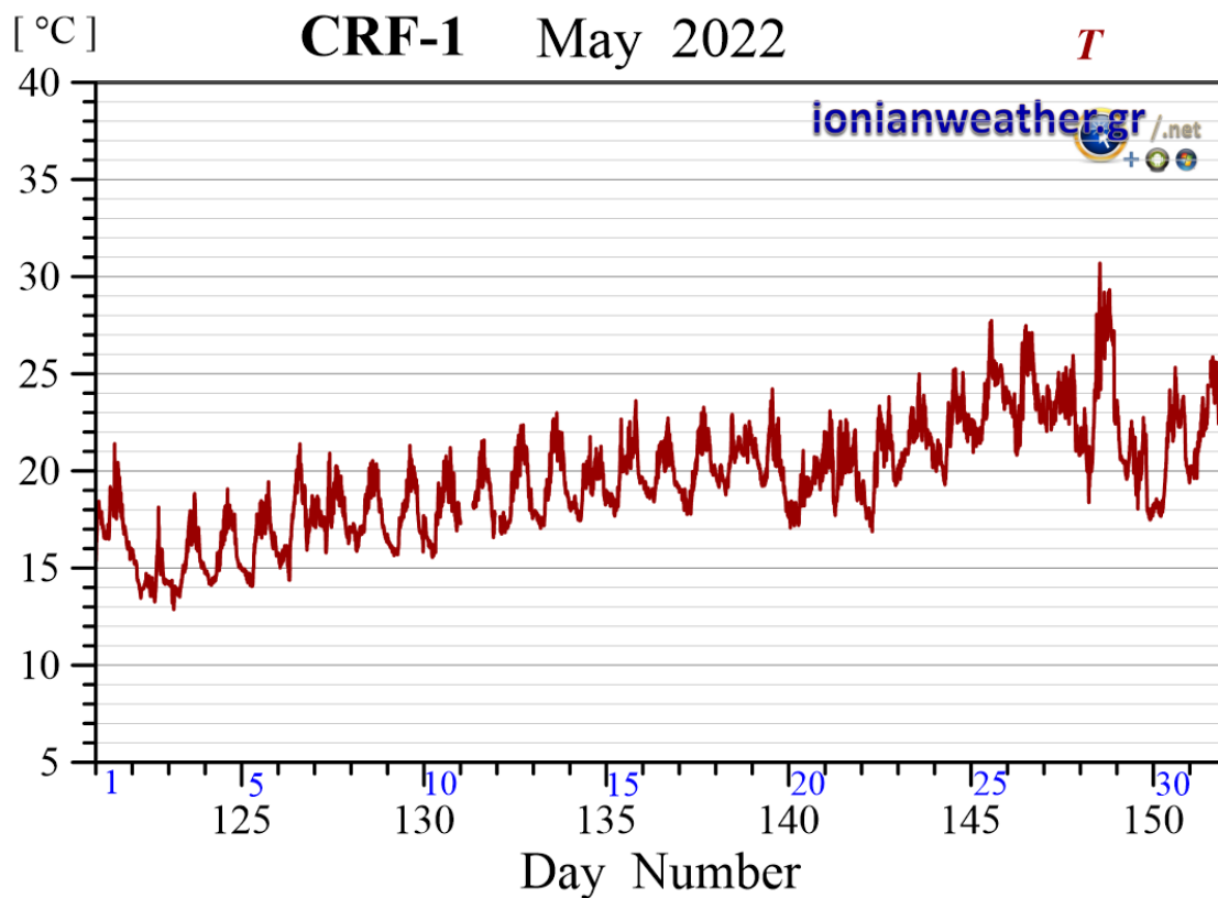
Εικόνα CRF1-4: Μέση ανά λεπτό θερμοκρασία αέρα Μαΐου 2022.
