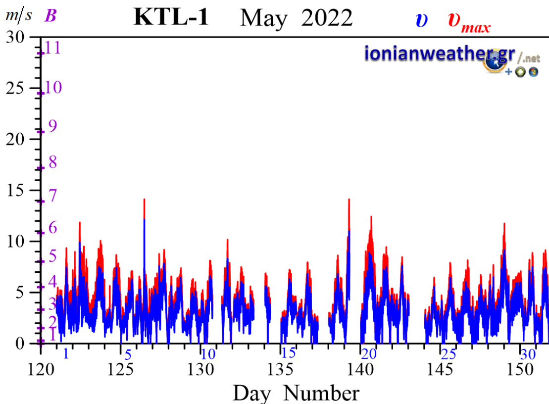
Εικόνα KTL1-2: Μέση ανά λεπτό ταχύτητα ανέμου ( m/s , γαλάζιο) και ριπή ανέμου (κόκκινο) Μαΐου 2022. Κλίμακα ταχυτήτων αριστερά σε m/s και Beaufort .
