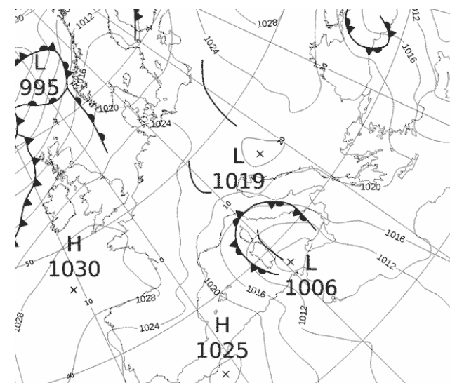
Εικόνα 3.1-6: MSLP 6 May 2022 00UTC
