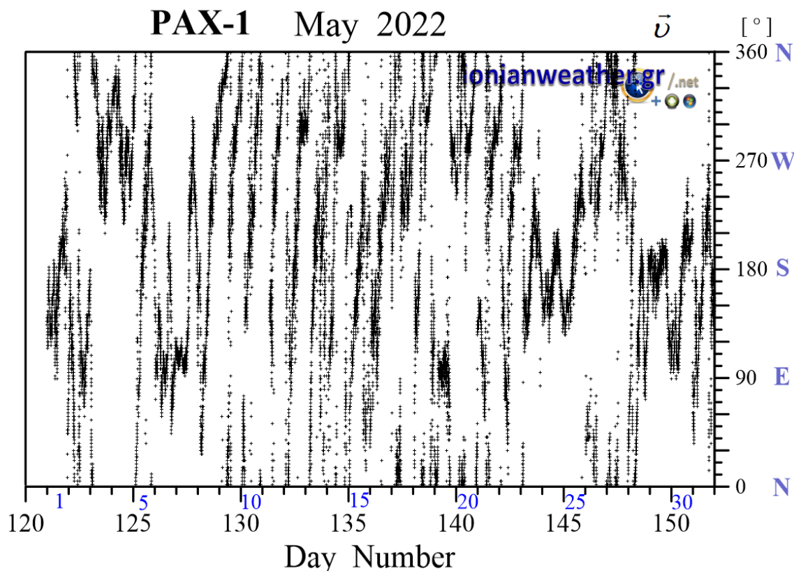
Εικόνα PAX 1-3: Μέση ανά λεπτό κατεύθυνση ανέμου Μαΐου 2022 (κλίμακα αζιμουθίων δεξιά)
