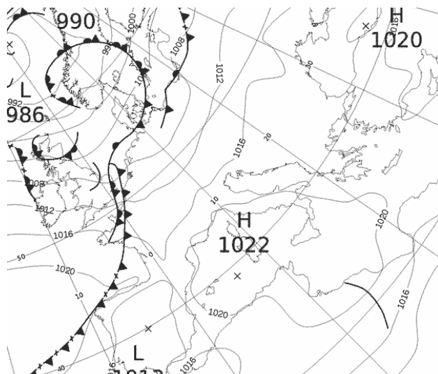
Εικόνα 3.1-12: MSLP 12 May 2022 00UTC
