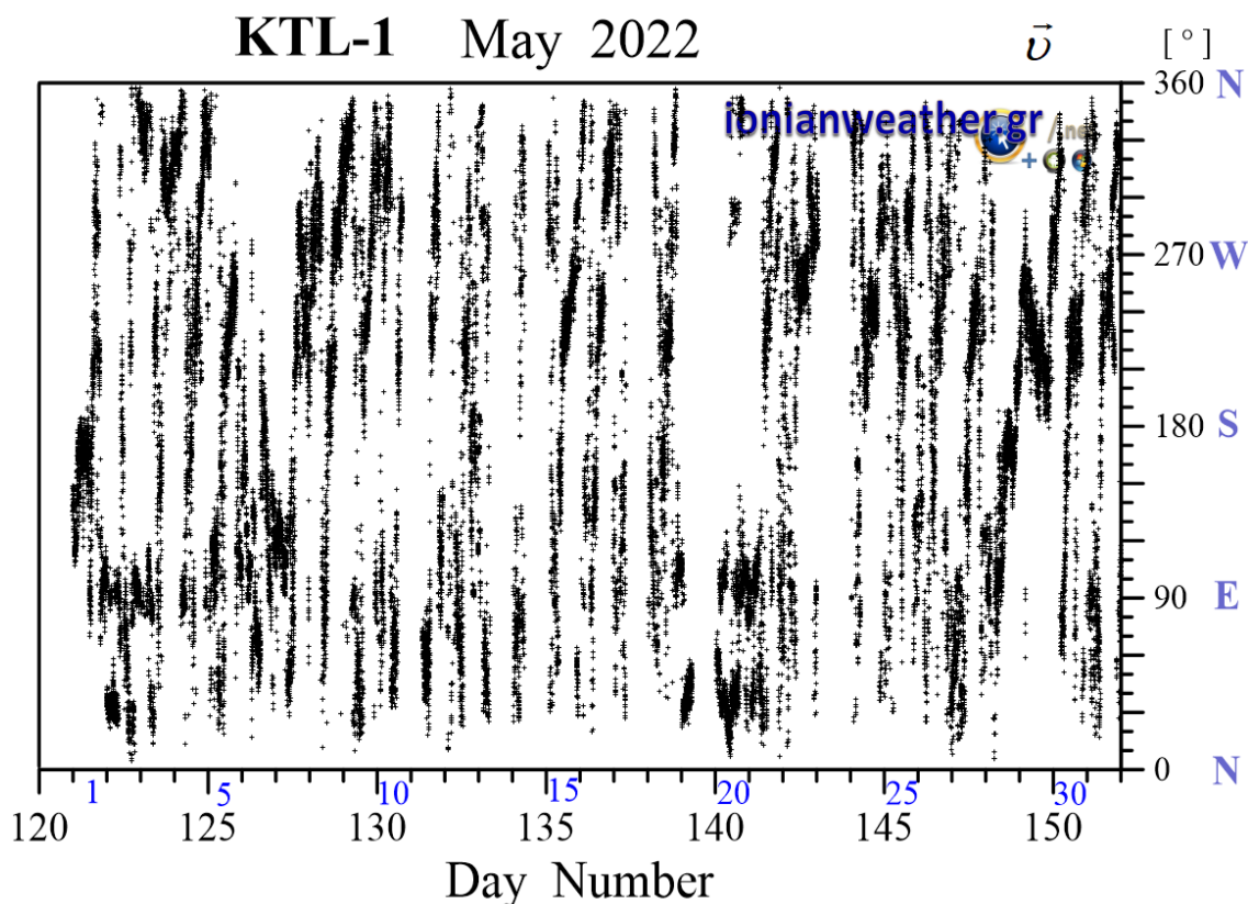
Εικόνα KTL1-3: Μέση ανά λεπτό κατεύθυνση ανέμου Μαΐου 2022 (κλίμακα αζιμουθίων δεξιά)
