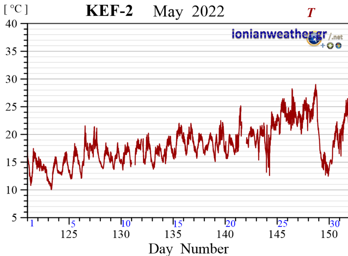
Εικόνα KEF2-4 Μέση ανά λεπτό θερμοκρασία αέρα Μαΐου 2022.
