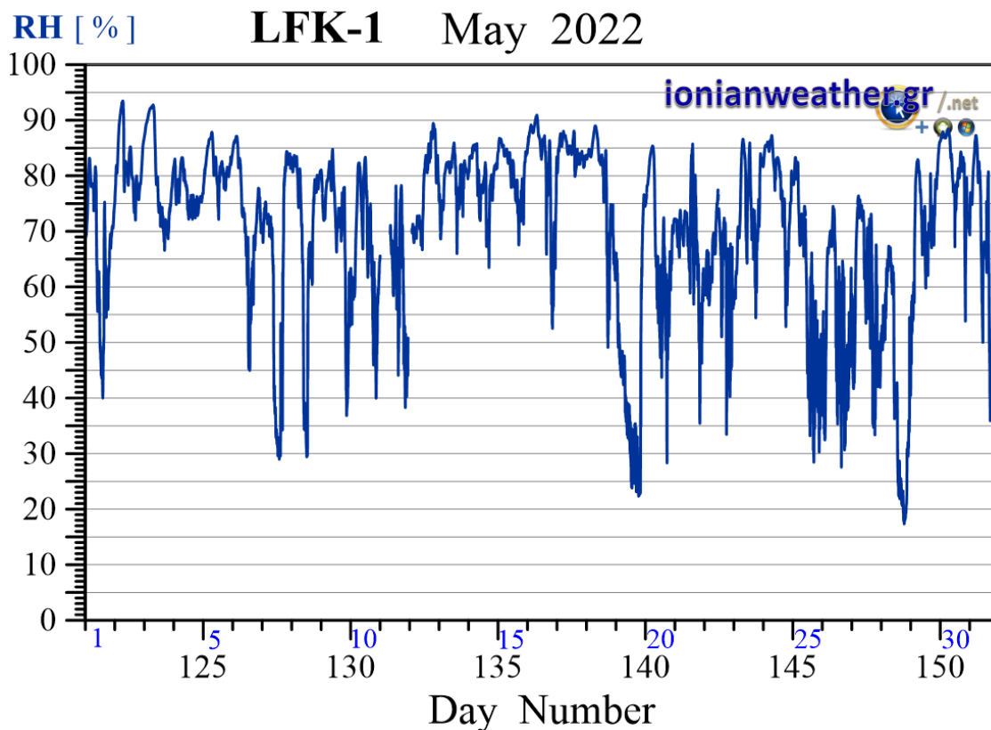
Εικόνα LFK1-5: Μέση ανά λεπτό σχετική υγρασία Μαΐου 2022.
