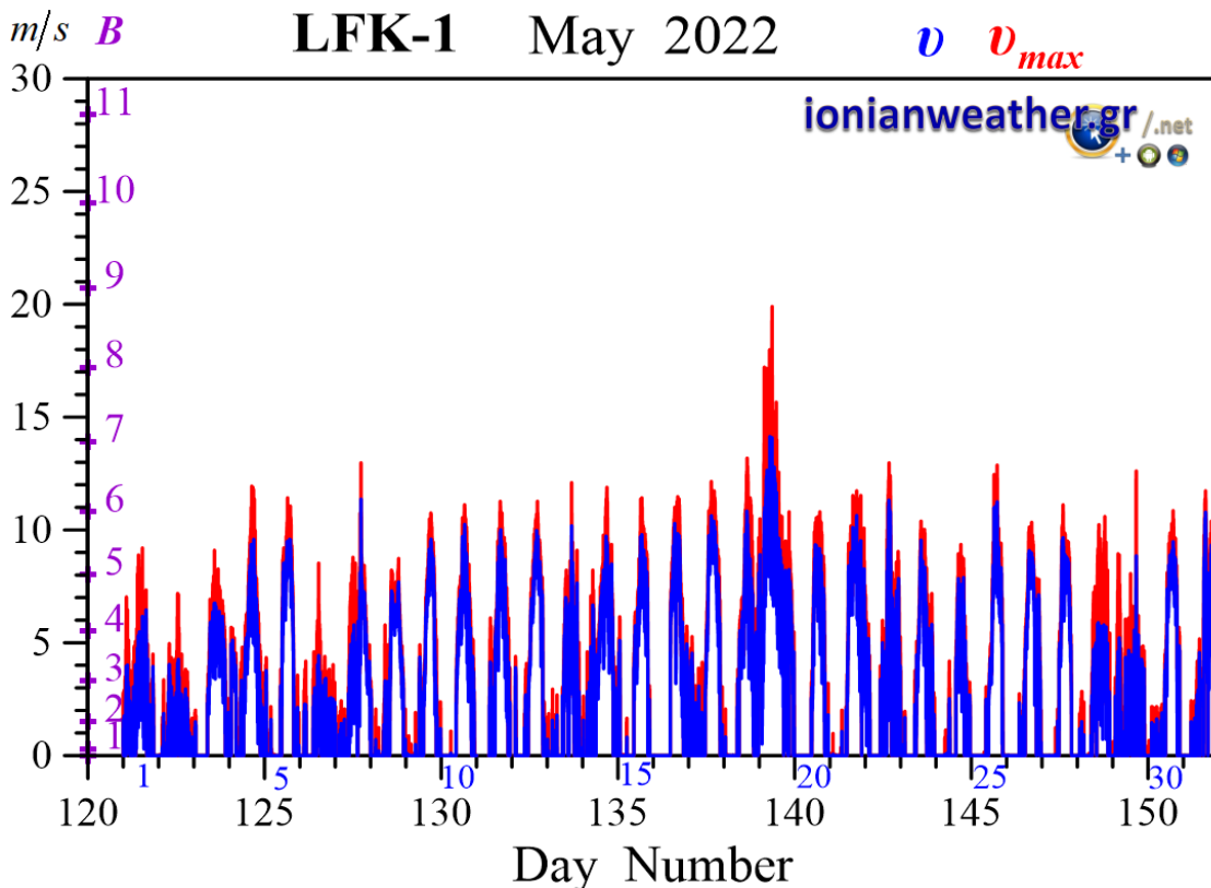
Εικόνα LFK1-2: Μέση ανά λεπτό ταχύτητα ανέμου (m/s, γαλάζιο) και ριπή ανέμου (κόκκινο) Μαΐου 2022. Κλίμακα ταχυτήτων αριστερά σε m/s και Beaufort.
