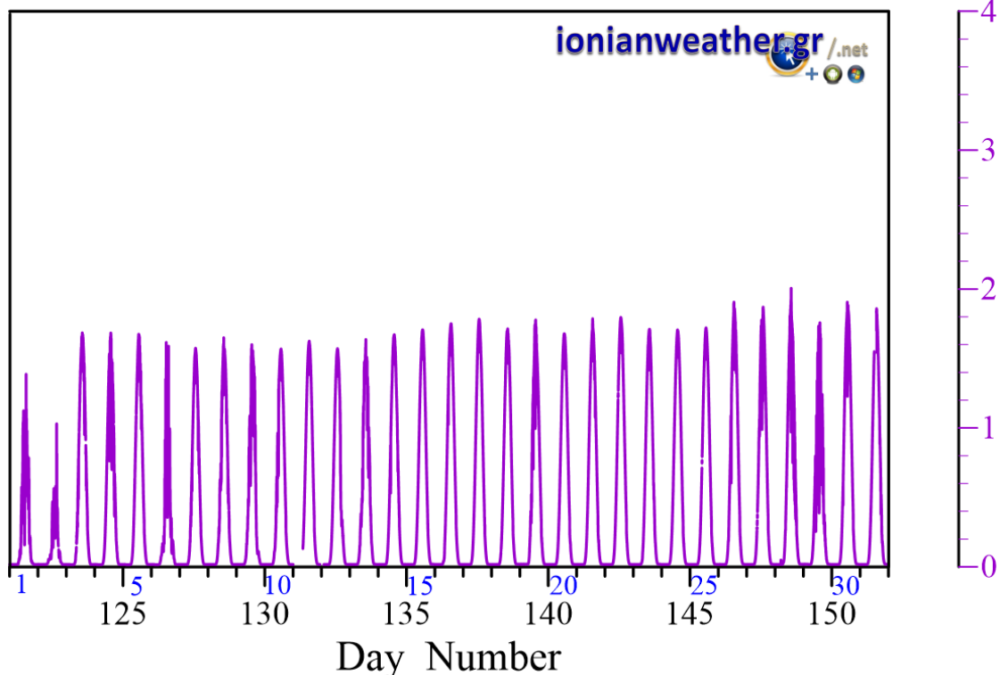
Εικόνα ZKT2-9: Μέση ανά λεπτό Ηλιακή ακτινοβολία Μαΐου 2022 στην φασματική περιοχή UVB
