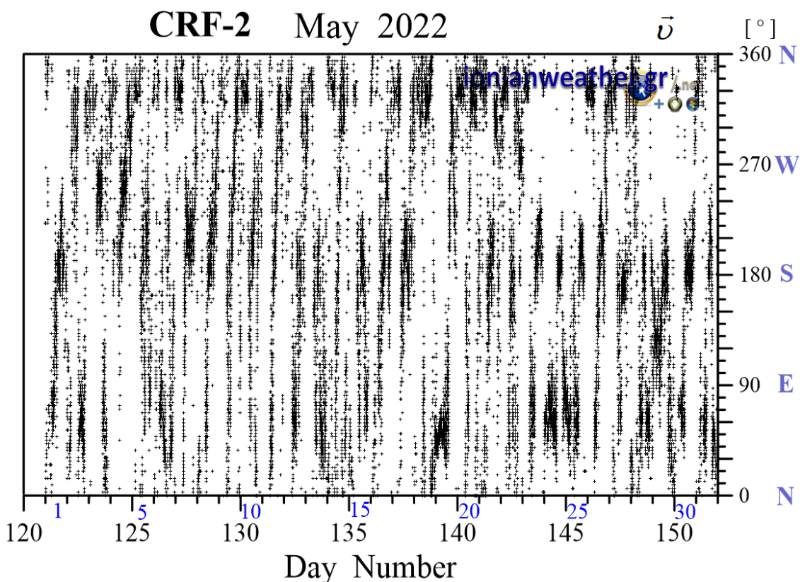
Εικόνα CRF2-3: Μέση ανά λεπτό κατεύθυνση ανέμου Μαΐου 2022 (κλίμακα αζιμουθίων δεξιά)
