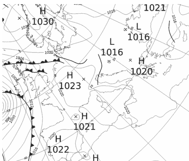
Εικόνα 3.1-17: MSLP 17 May 2022 00UTC
