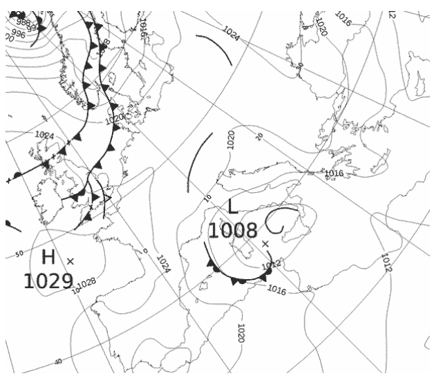
Εικόνα 3.1-7: MSLP 7 May 2022 00UTC
