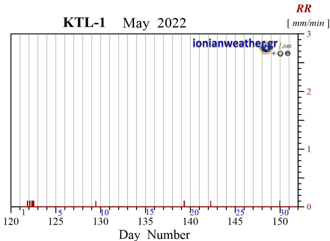
Εικόνα KTL1-1: Ανά λεπτό ρυθμός βροχόπτωσης (mm/min) Μαΐου 2022.
