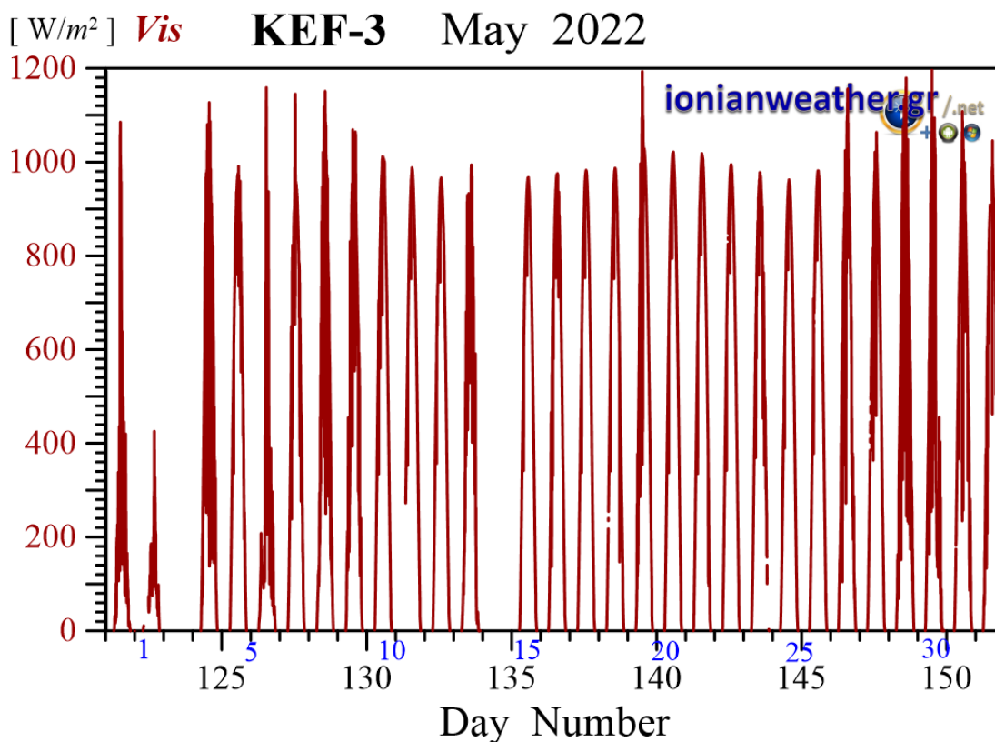
Εικόνα KEF3-7: Μέση ανά λεπτό Ηλιακή ακτινοβολία Μαΐου 2022 στην οπτική και εγγύς υπέρυθρη περιοχή.
