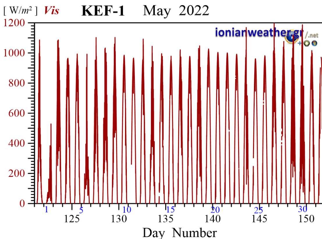
Εικόνα KEF1-7: Μέση ανά λεπτό Ηλιακή ακτινοβολία Μαΐου 2022 στην οπτική και εγγύς υπέρυθρη περιοχή.
