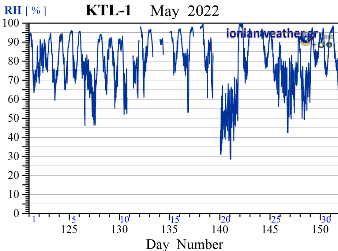
Εικόνα KTL1-5: Μέση ανά λεπτό σχετική υγρασία Μαΐου 2022.
