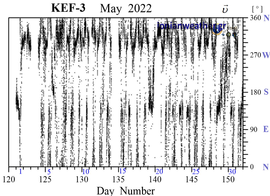
Εικόνα KEF3-3: Μέση ανά λεπτό κατεύθυνση ανέμου Μαΐου 2022 (κλίμακα αζιμουθίων δεξιά)
