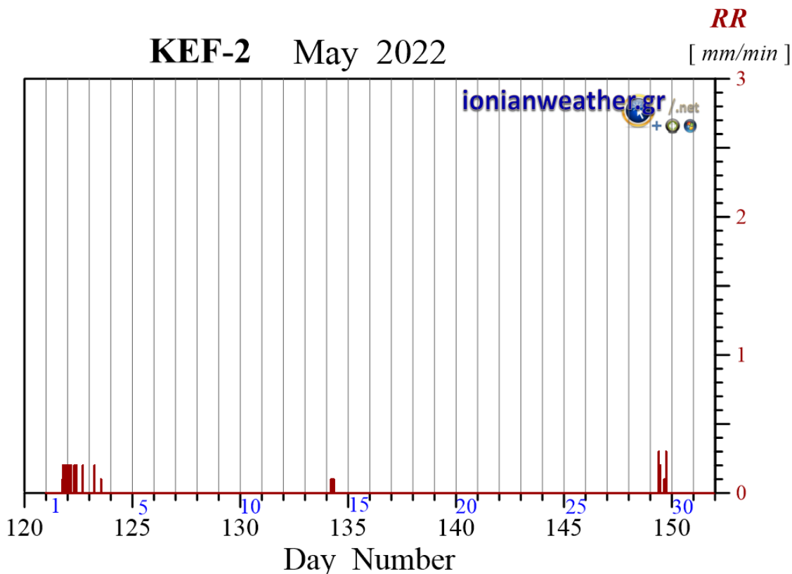
Εικόνα KEF2-1: Ανά λεπτό ρυθμός βροχόπτωσης (mm/min) Μαΐου 2022.
