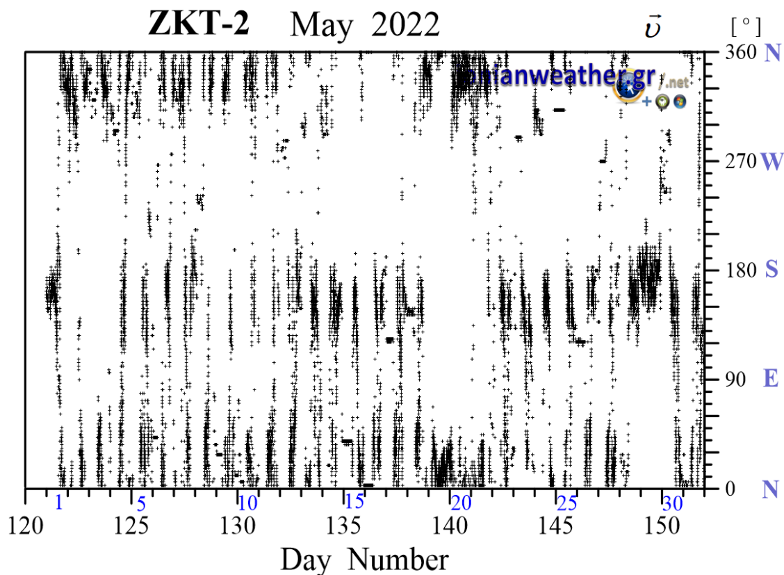
Εικόνα ZKT2-3: Μέση ανά λεπτό κατεύθυνση ανέμου Μαΐου 2022 (κλίμακα αζιμουθίων δεξιά)
