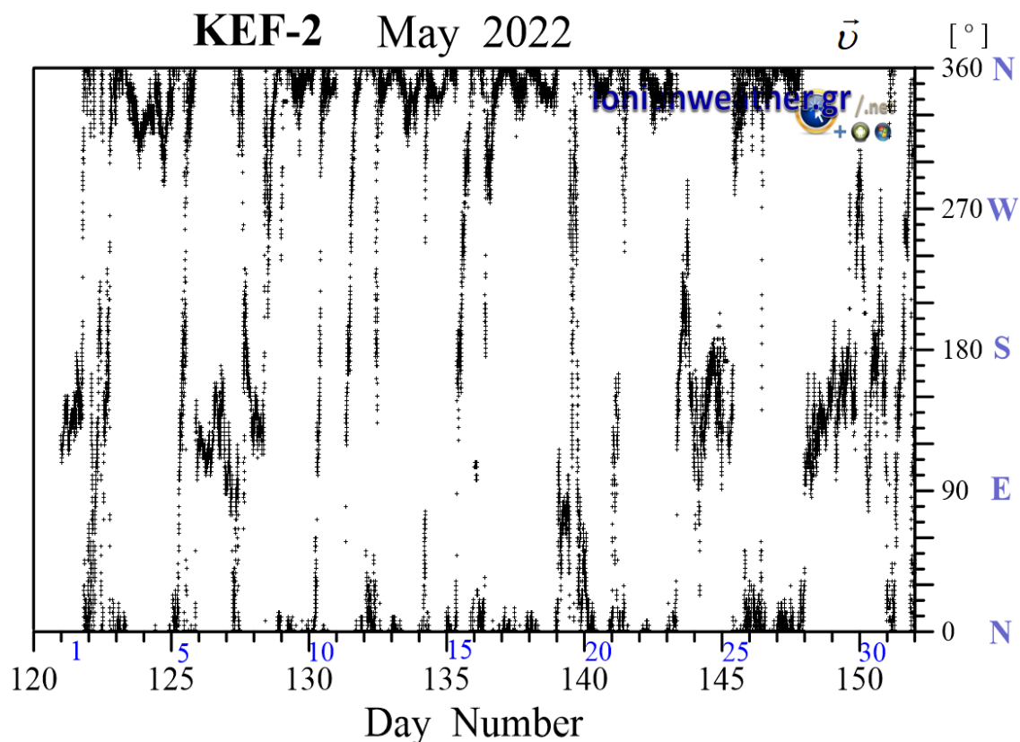
Εικόνα KEF2-3: Μέση ανά λεπτό κατεύθυνση ανέμου Μαΐου 2022 (κλίμακα αζιμουθίων δεξιά)
