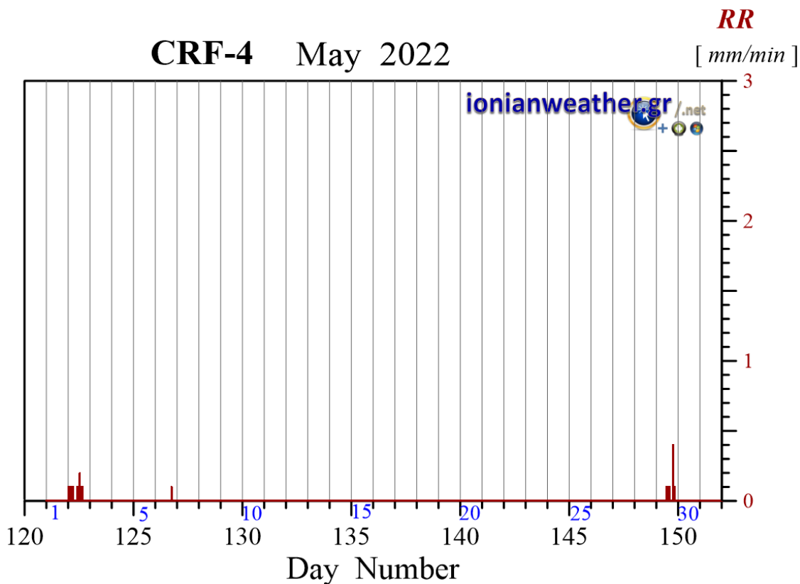
Εικόνα CRF4-1: Ανά λεπτό ρυθμός βροχόπτωσης (mm/min) Μαΐου 2022.
