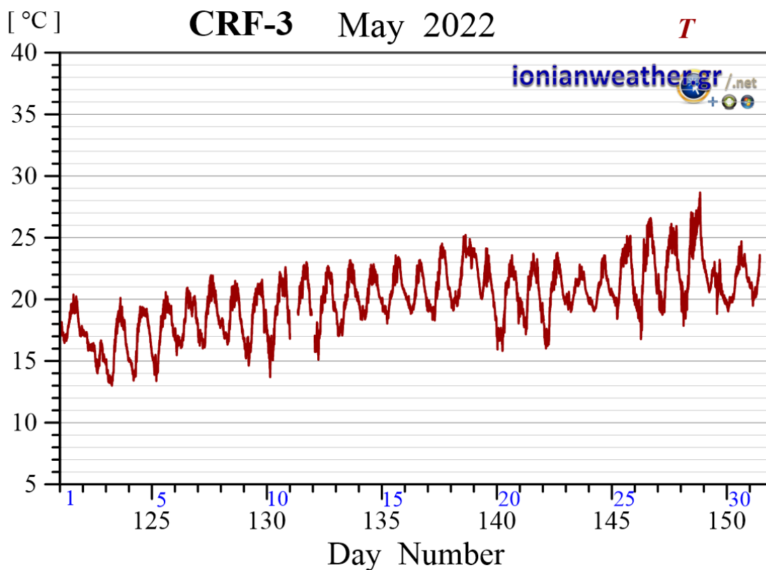
Εικόνα CRF3-4: Μέση ανά λεπτό θερμοκρασία αέρα Μαΐου 2022.
