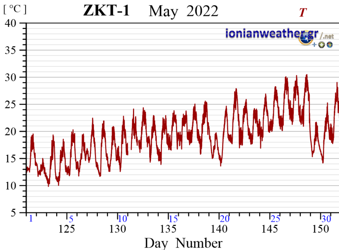
Εικόνα ZKT1-4: Μέση ανά λεπτό θερμοκρασία αέρα Μαΐου 2022.
