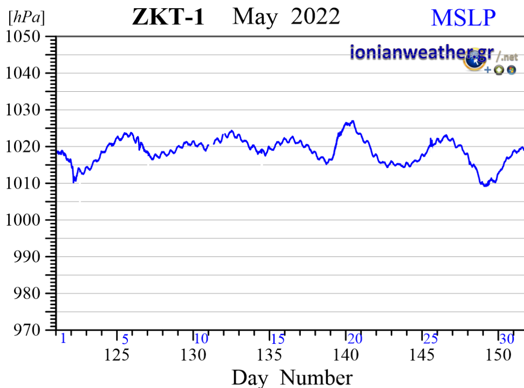
Εικόνα ZKT1-6: Μέση ανά λεπτό βαρομετρική πίεση Μαΐου 2022 ανηγμένη στην επιφάνεια της θάλασσας.
