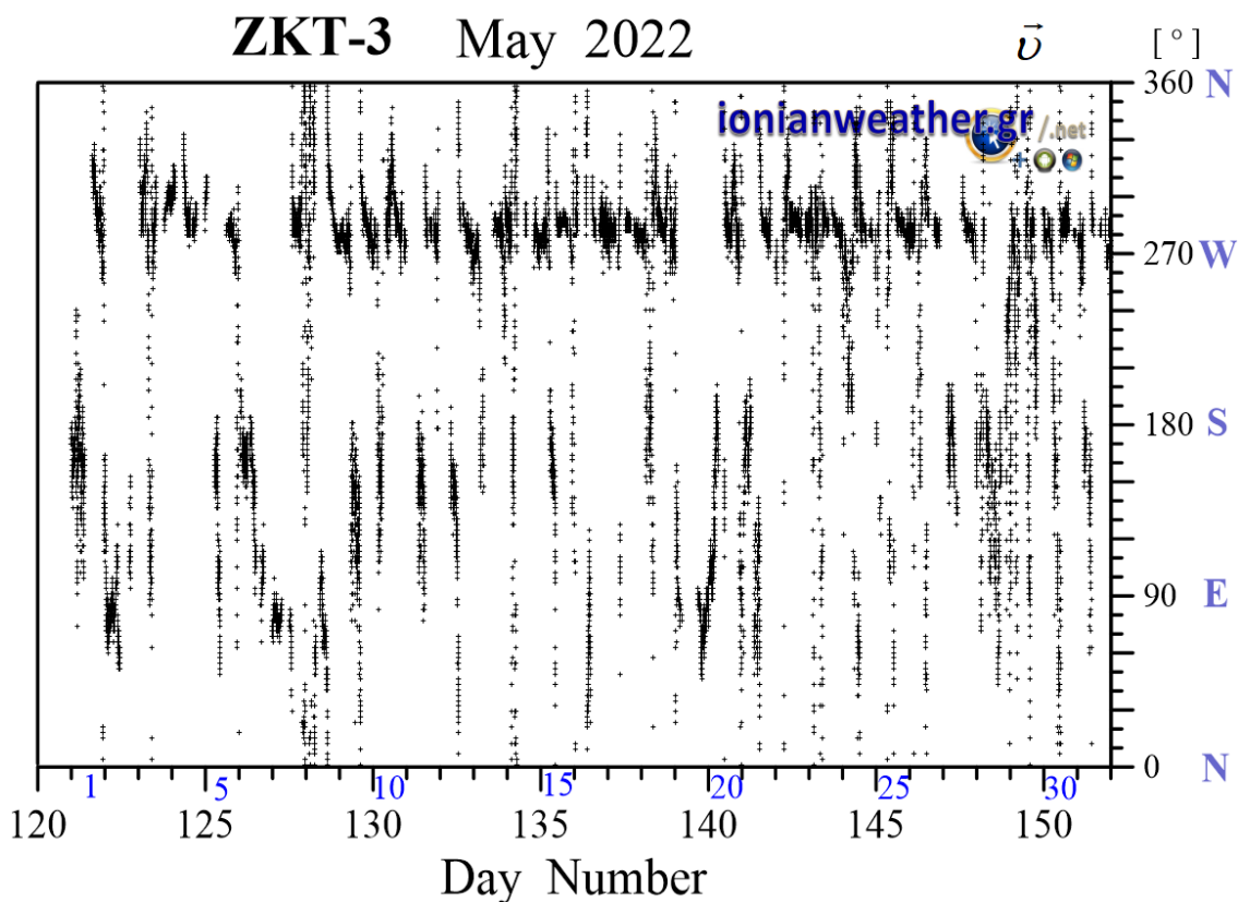
Εικόνα ZKT3-3: Μέση ανά λεπτό κατεύθυνση ανέμου Μαΐου 2022 (κλίμακα αζιμουθίων δεξιά)
