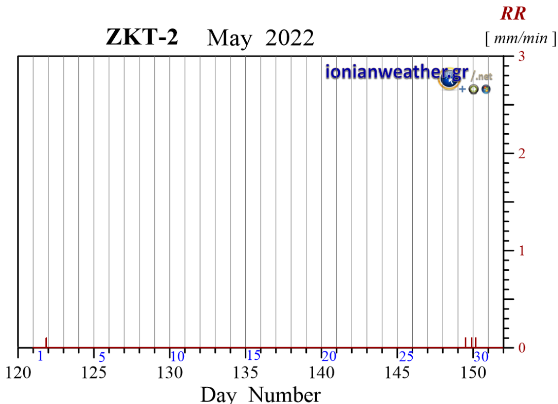
Εικόνα ZKT2-1: Ανά λεπτό ρυθμός βροχόπτωσης (mm/min) Μαΐου 2022.
