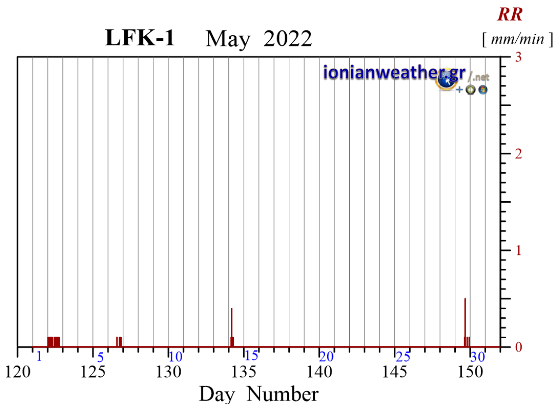
Εικόνα LFK1-1: Ανά λεπτό ρυθμός βροχόπτωσης (mm/min) Μαΐου 2022.
