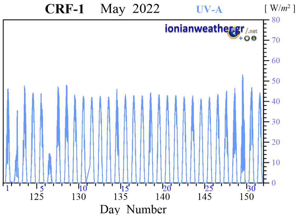
Εικόνα CRF1-8: Μέση ανά λεπτό Ηλιακή ακτινοβολία Μαΐου 2022 στη φασματική περιοχή UVA.
