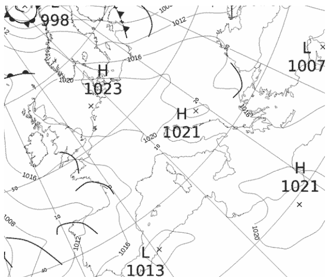
Εικόνα 3.1-15: MSLP 15 May 2022 00UTC
