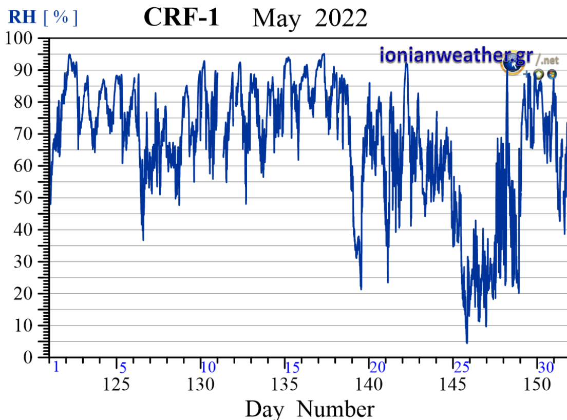
Εικόνα CRF1-5: Μέση ανά λεπτό σχετική υγρασία Μαΐου 2022.
