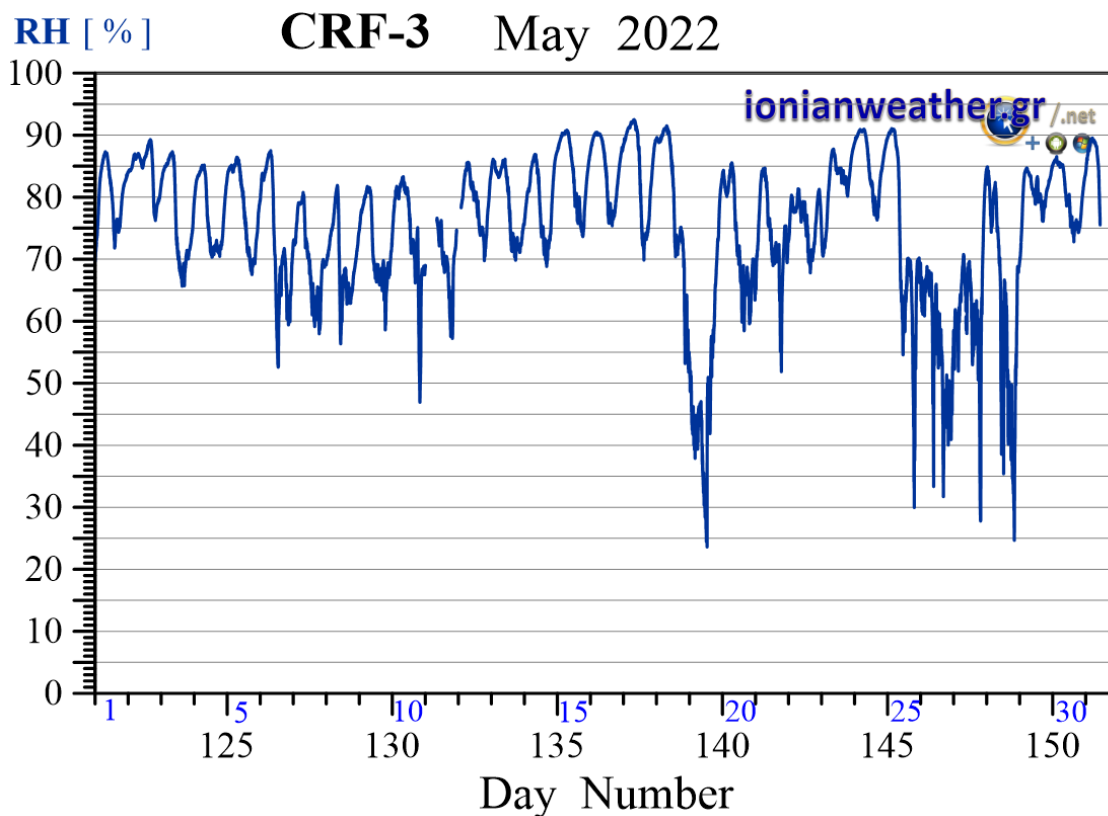
Εικόνα CRF3-5: Μέση ανά λεπτό σχετική υγρασία Μαΐου 2022.
