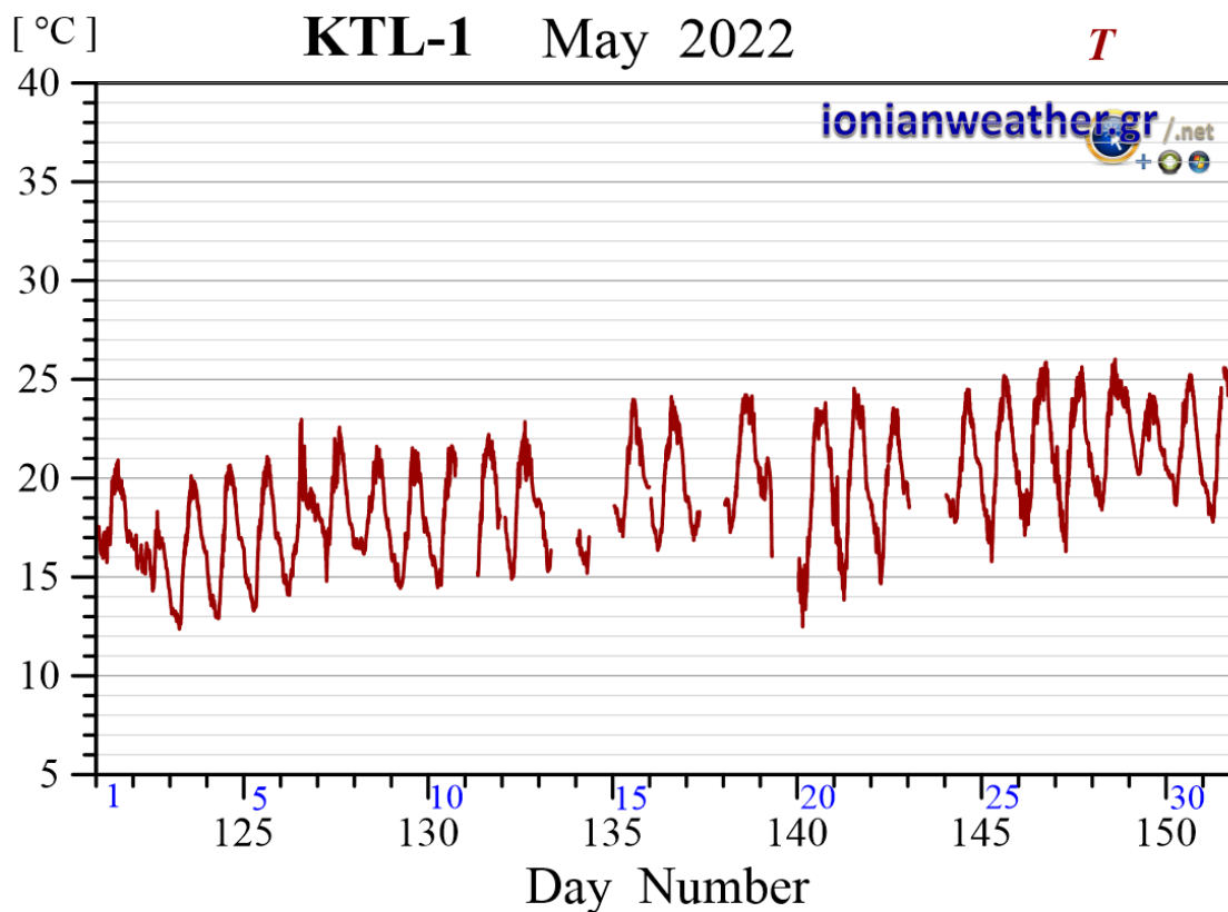
Εικόνα KTL1-4: Μέση ανά λεπτό θερμοκρασία αέρα Μαΐου 2022.
