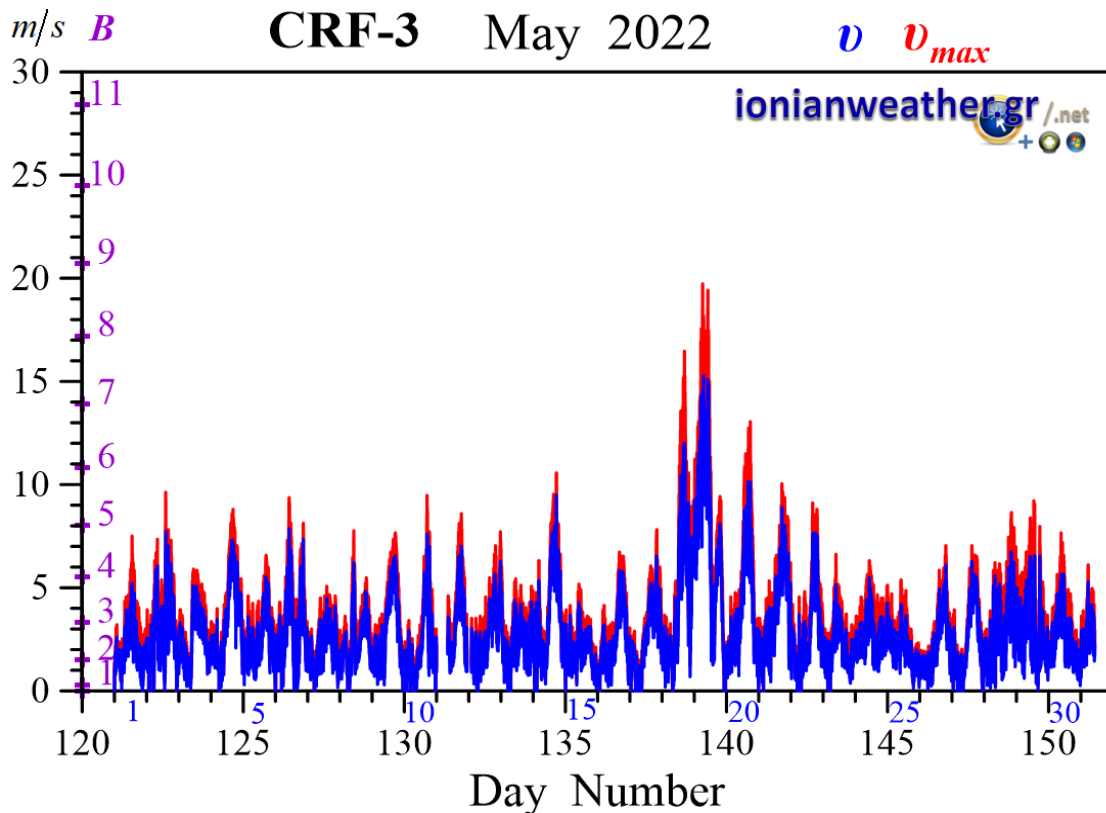
Εικόνα CRF3-2: Μέση ανά λεπτό ταχύτητα ανέμου (m/s, γαλάζιο) και ριπή ανέμου (κόκκινο) Μαΐου 2022. Κλίμακα ταχυτήτων αριστερά σε m/s και Beaufort.
