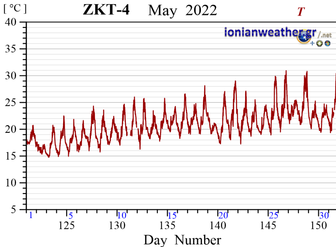
Εικόνα ZKT4-4: Μέση ανά λεπτό θερμοκρασία αέρα Μαΐου 2022.
