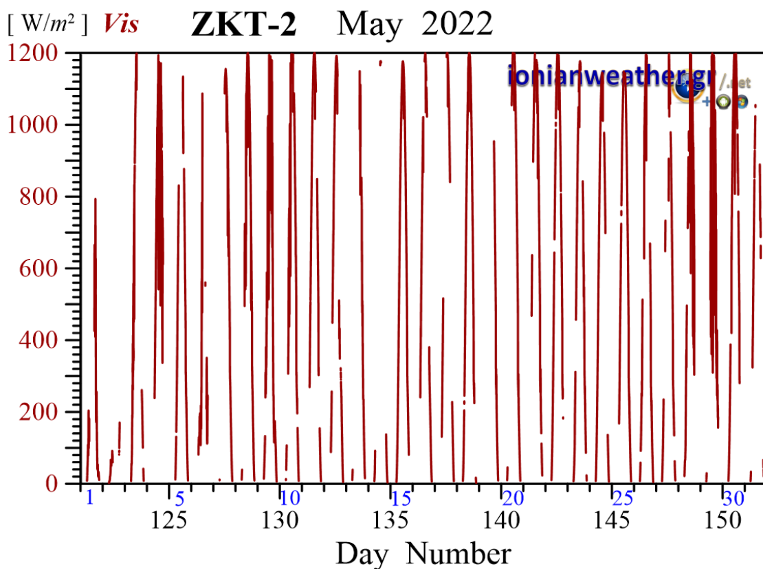
Εικόνα ZKT2-7: Μέση ανά λεπτό Ηλιακή ακτινοβολία Μαΐου 2022 στην οπτική και εγγύς υπέρυθρη περιοχή.
