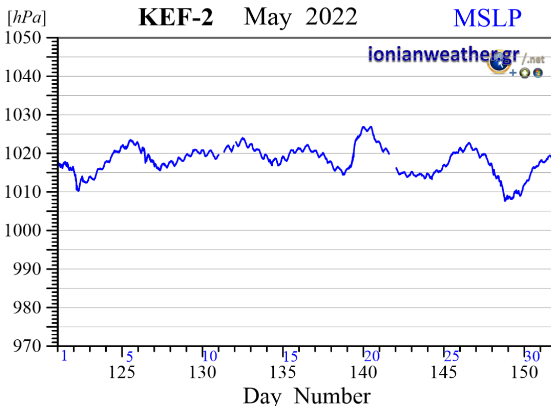
Εικόνα KEF2-6: Μέση ανά λεπτό βαρομετρική πίεση Μαΐου 2022 ανηγμένη στην επιφάνεια της θάλασσας.
