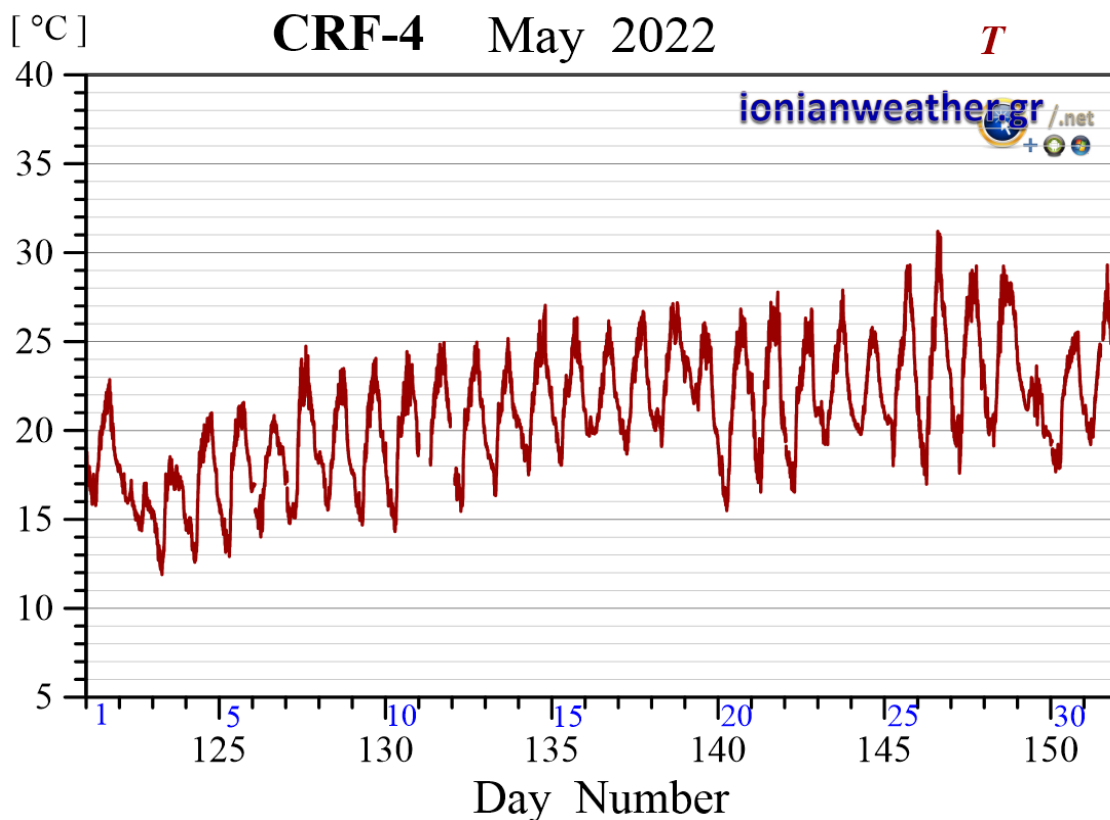
Εικόνα CRF4-4: Μέση ανά λεπτό θερμοκρασία αέρα Μαΐου 2022.
