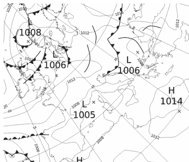
Εικόνα 3.1-30: MSLP 30 May 2022 00UTC
