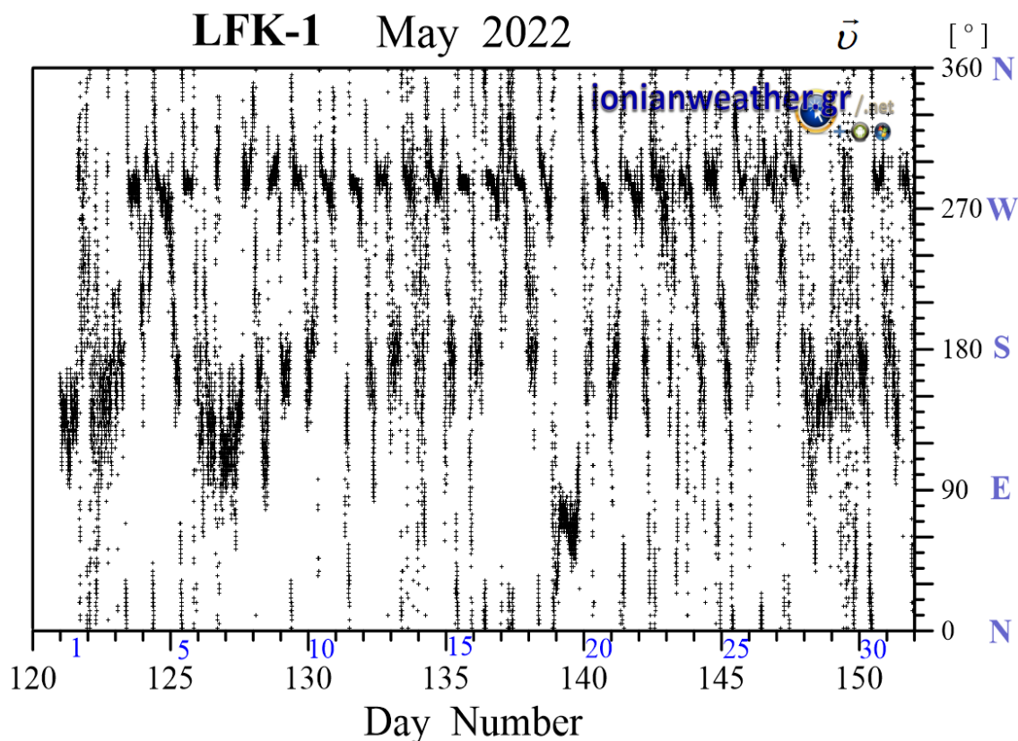
Εικόνα LFK1-3: Μέση ανά λεπτό κατεύθυνση ανέμου Μαΐου 2022 (κλίμακα αζιμουθίων δεξιά)
