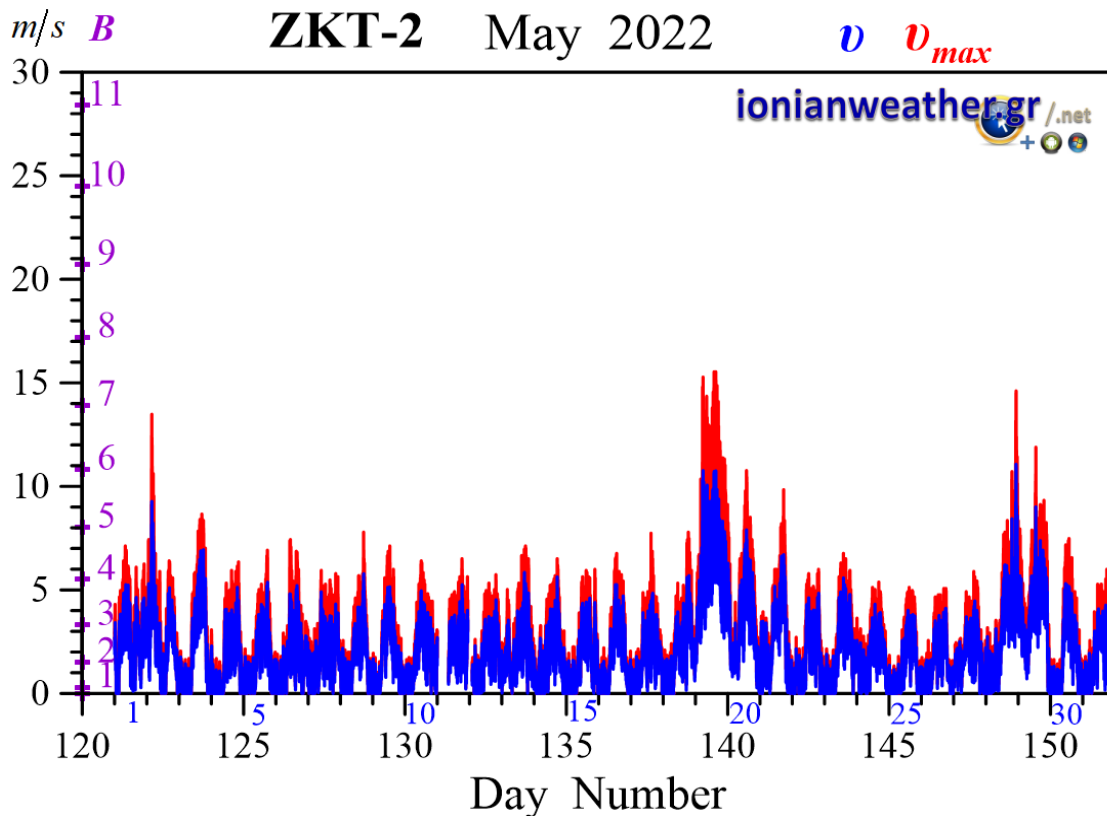
Εικόνα ZKT2-2: Μέση ανά λεπτό ταχύτητα ανέμου (m/s, γαλάζιο) και ριπή ανέμου (κόκκινο) Μαΐου 2022. Κλίμακα ταχυτήτων αριστερά σε m/s και Beaufort.
