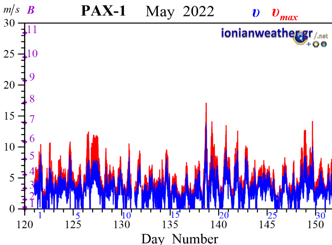
Εικόνα PAX 1-2: Μέση ανά λεπτό ταχύτητα ανέμου (m/s, γαλάζιο) και ριπή ανέμου (κόκκινο) Μαΐου 2022. Κλίμακα ταχυτήτων αριστερά σε m/s και Beaufort.
