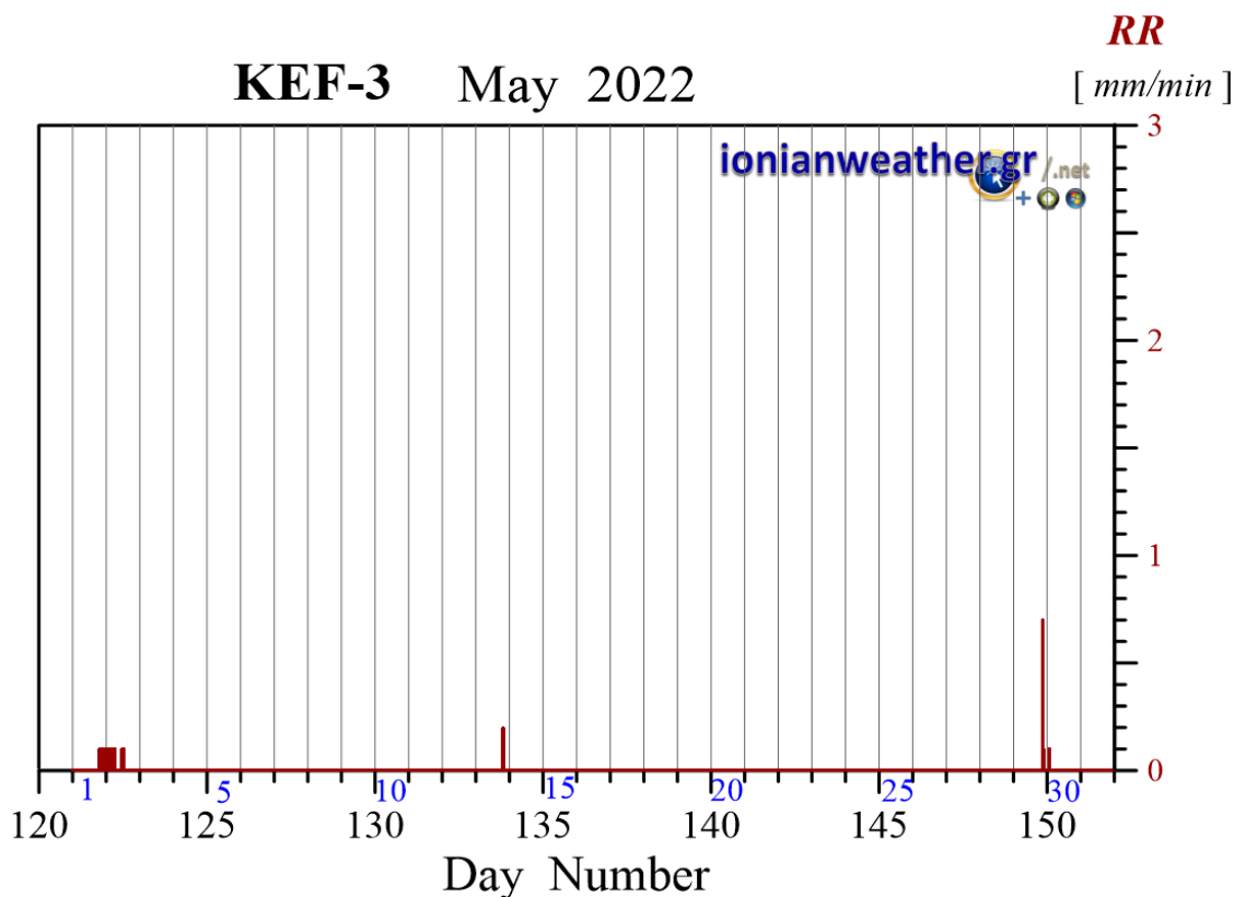
Εικόνα KEF3-1: Ανά λεπτό ρυθμός βροχόπτωσης (mm/min) Μαΐου 2022.
