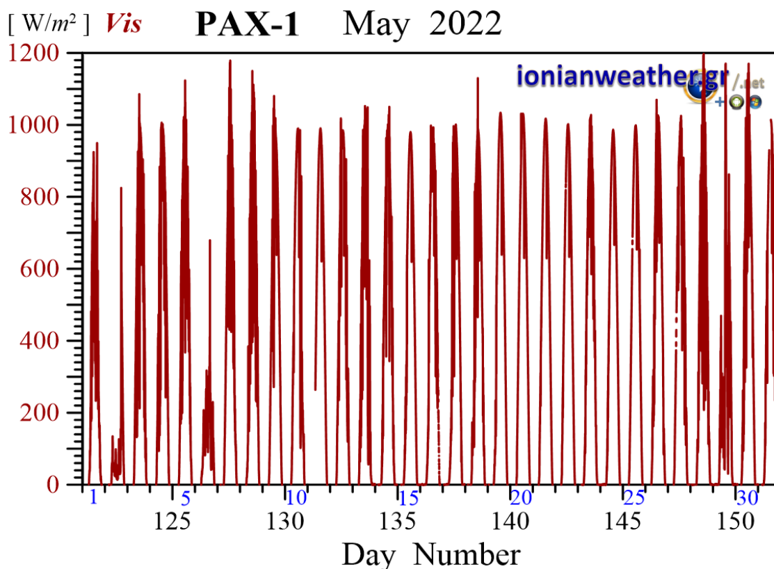
Εικόνα PAX1-6: Μέση ανά λεπτό Ηλιακή ακτινοβολία Μαΐου 2022 στην οπτική και εγγύς υπέρυθρη περιοχή.
