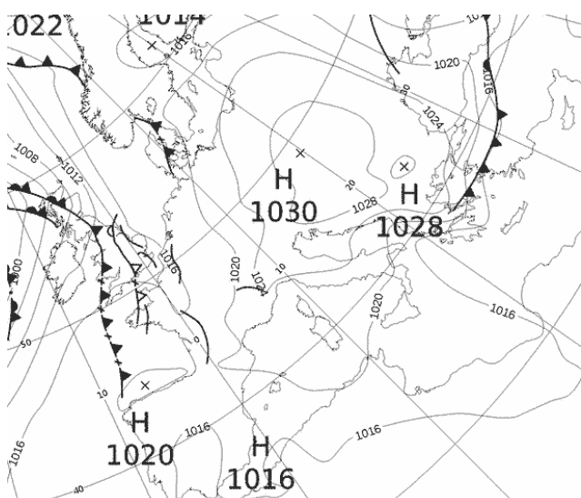
Εικόνα 3.1-19: MSLP 19 May 2022 00UTC
