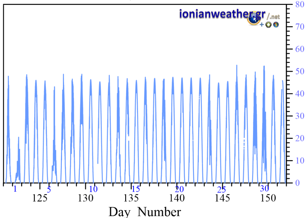
Εικόνα KEF1-8: Μέση ανά λεπτό Ηλιακή ακτινοβολία Μαΐου 2022 στη φασματική περιοχή UVA.
