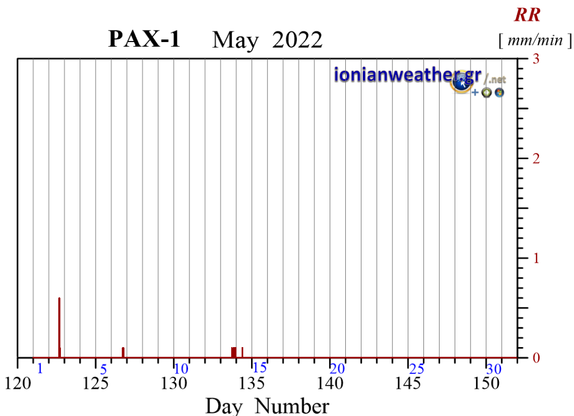
Εικόνα PAX1-1: Ανά λεπτό ρυθμός βροχόπτωσης (mm/min) Μαΐου 2022.
