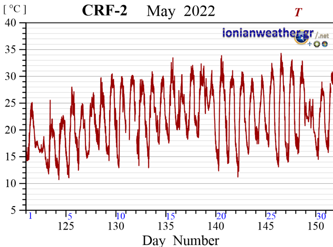
Εικόνα CRF2-4: Μέση ανά λεπτό θερμοκρασία αέρα Μαΐου 2022.
