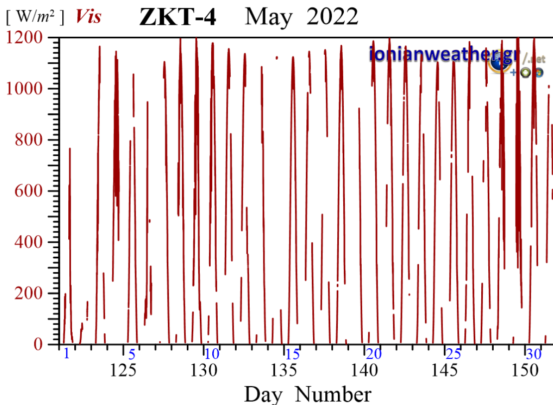
Εικόνα ZKT4-7: Μέση ανά λεπτό Ηλιακή ακτινοβολία Μαΐου 2022 στην οπτική και εγγύς υπέρυθρη περιοχή.
