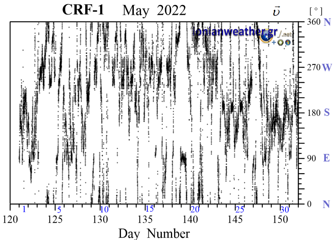
Εικόνα CRF1-3: Μέση ανά λεπτό κατεύθυνση ανέμου Μαΐου 2022 (κλίμακα αζιμουθίων δεξιά)
