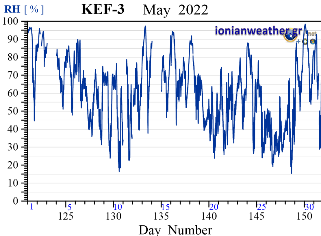
Εικόνα KEF3-5: Μέση ανά λεπτό σχετική υγρασία Μαΐου 2022.
