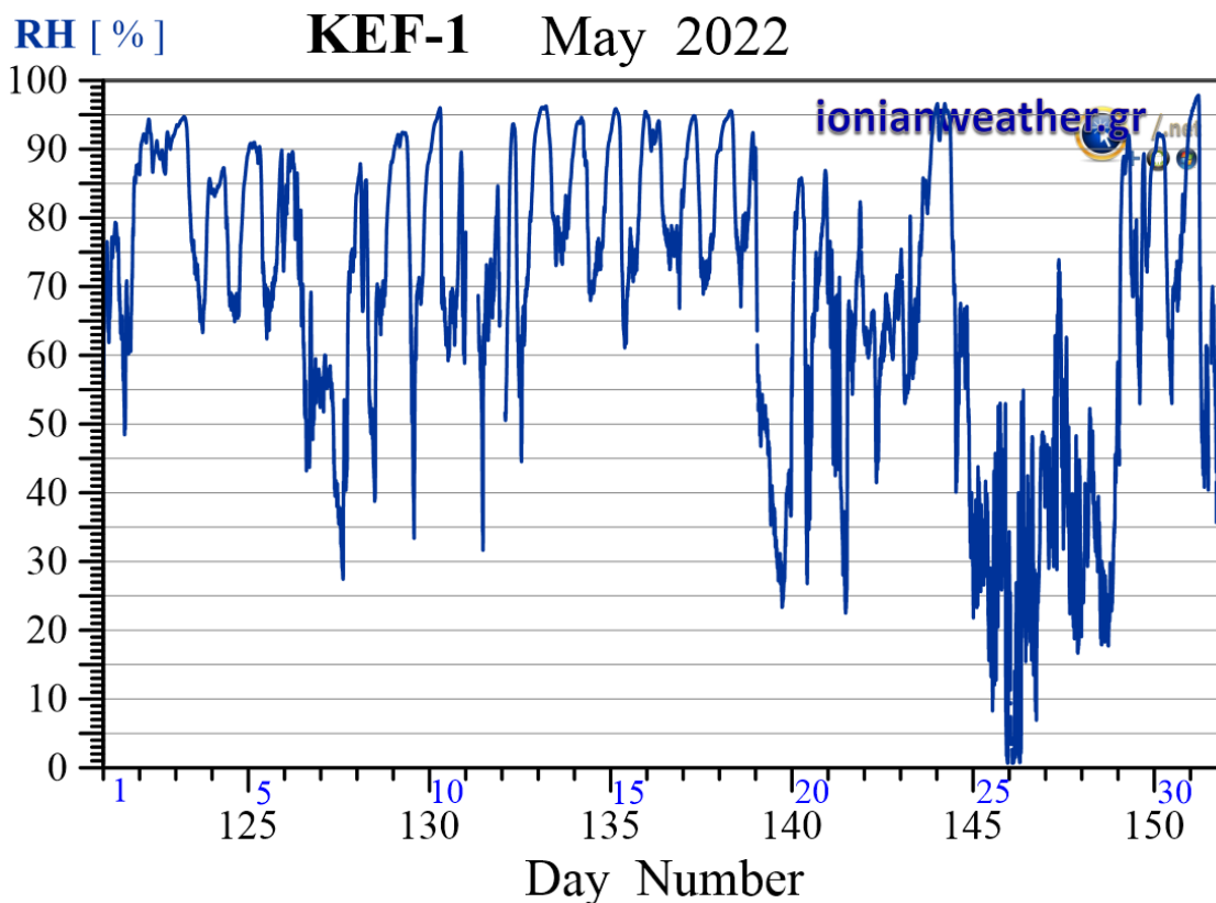
Εικόνα KEF1-5: Μέση ανά λεπτό σχετική υγρασία Μαΐου 2022.
