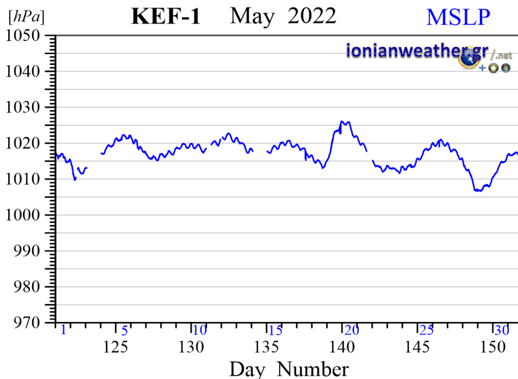
Εικόνα KEF1-6: Μέση ανά λεπτό βαρομετρική πίεση Μαΐου 2022 ανηγμένη στην επιφάνεια της θάλασσας.
