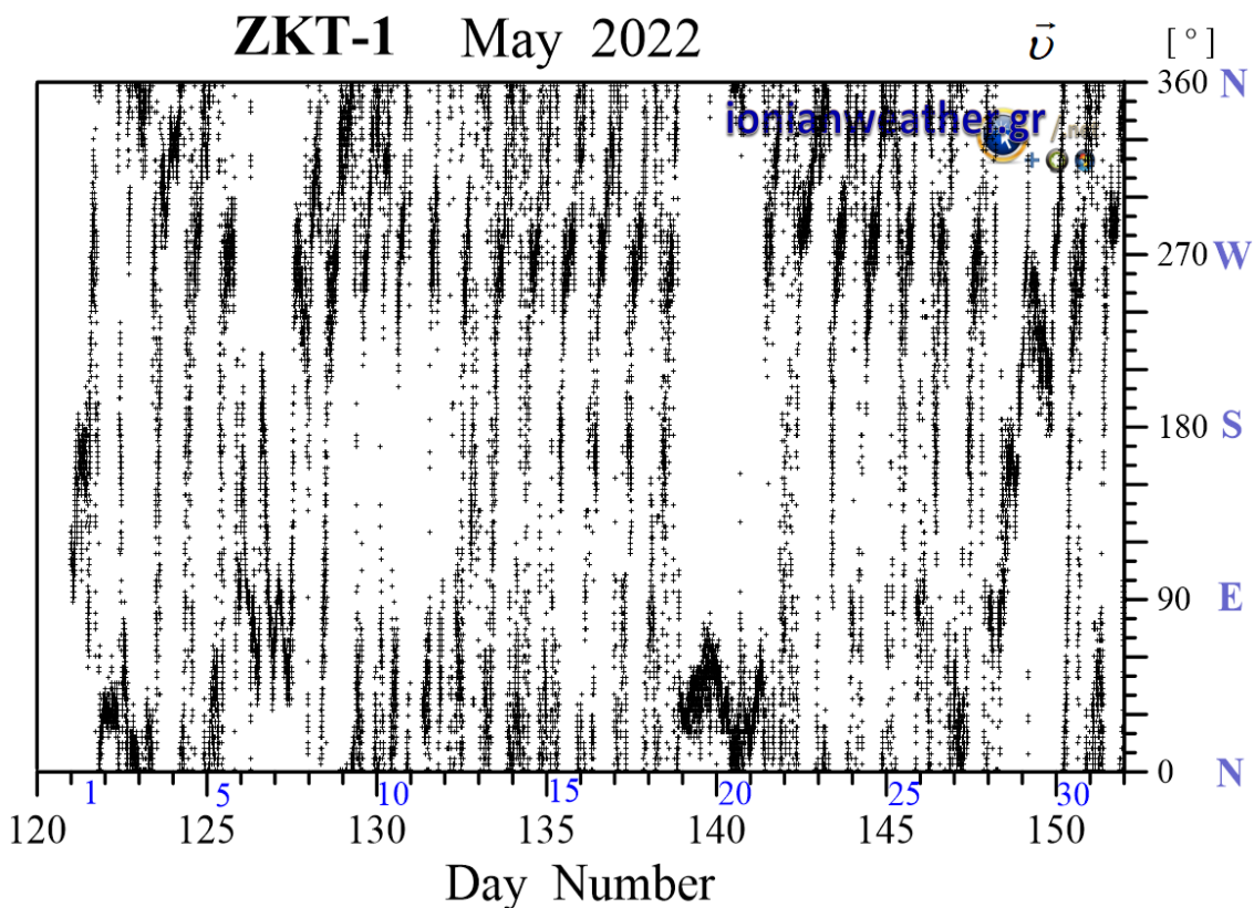
Εικόνα ZKT1-3: Μέση ανά λεπτό κατεύθυνση ανέμου Μαΐου 2022 (κλίμακα αζιμουθίων δεξιά)
