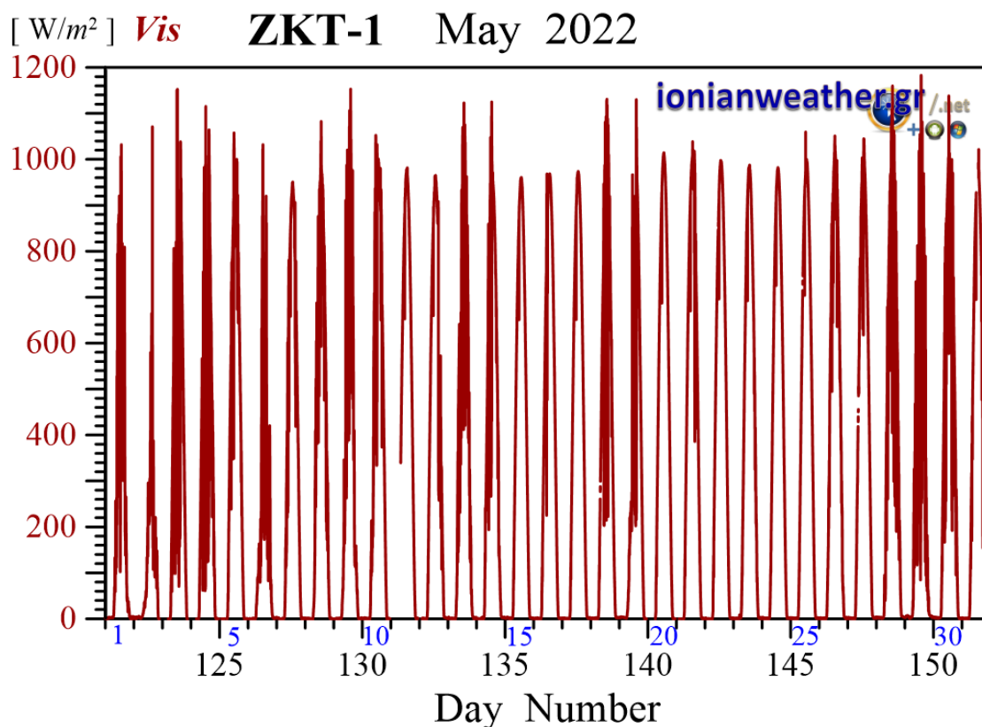
Εικόνα ZKT1-7: Μέση ανά λεπτό Ηλιακή ακτινοβολία Μαΐου 2022 στην οπτική και εγγύς υπέρυθρη περιοχή.
