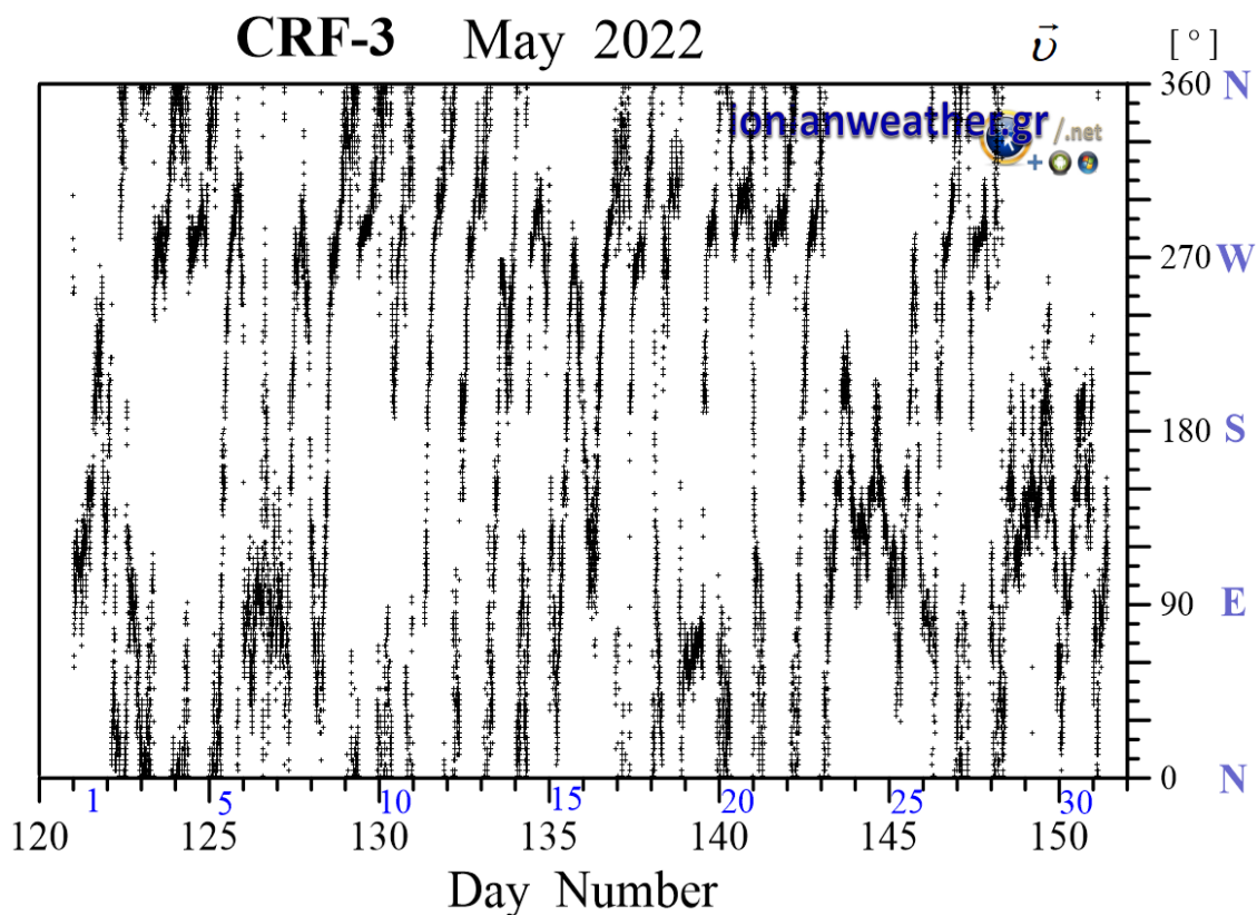
Εικόνα CRF3-3: Μέση ανά λεπτό κατεύθυνση ανέμου Μαΐου 2022 (κλίμακα αζιμουθίων δεξιά)
