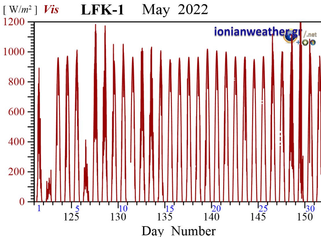
Εικόνα LFK1-7: Μέση ανά λεπτό Ηλιακή ακτινοβολία Μαΐου 2022 στην οπτική και εγγύς υπέρυθρη περιοχή.
