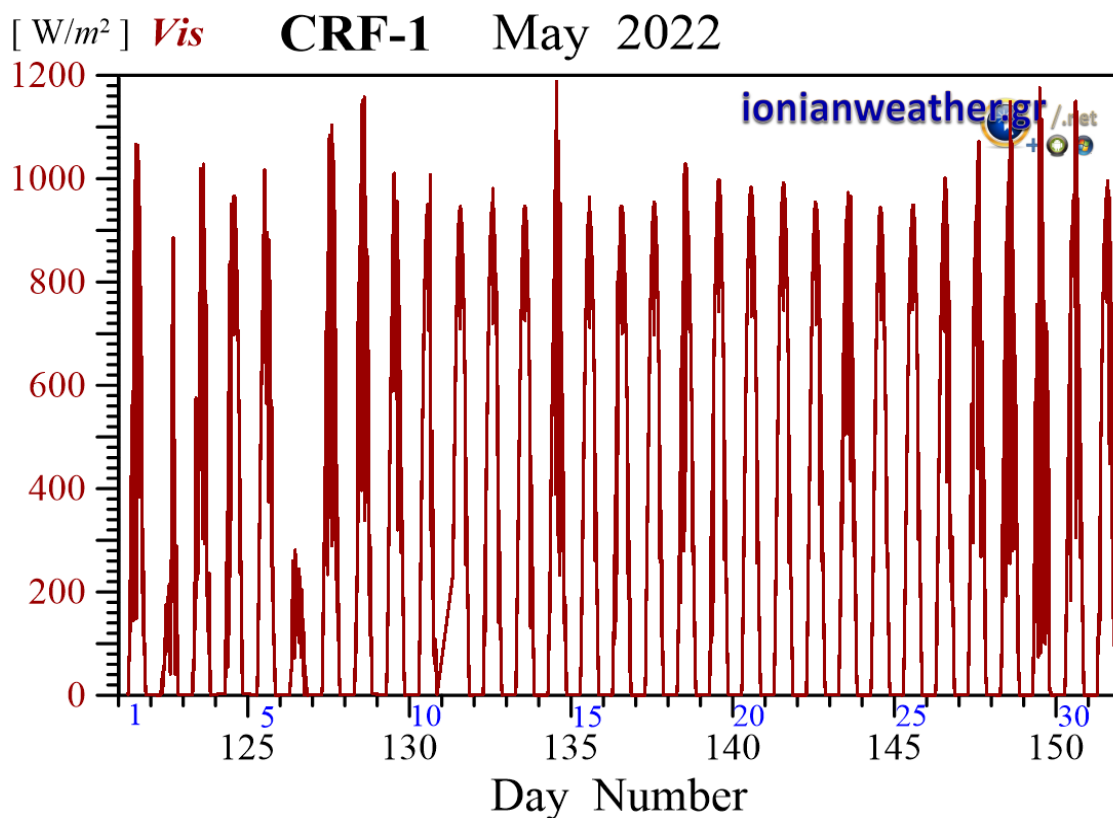
Εικόνα CRF1-7: Μέση ανά λεπτό Ηλιακή ακτινοβολία Μαΐου 2022 στην οπτική και εγγύς υπέρυθρη περιοχή.
