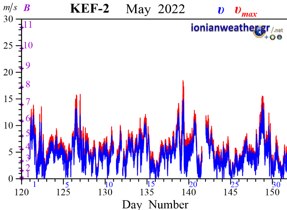
Εικόνα KEF2-2: Μέση ανά λεπτό ταχύτητα ανέμου (m/s, γαλάζιο) και ριπή ανέμου (κόκκινο) Μαΐου 2022. Κλίμακα ταχυτήτων αριστερά σε m/s και Beaufort.
