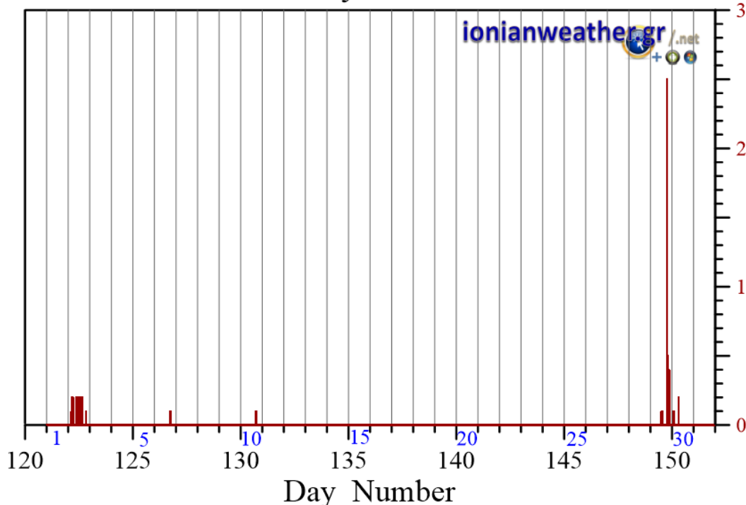
Εικόνα CRF2-1: Ανά λεπτό ρυθμός βροχόπτωσης (mm/min) Μαΐου 2022.
