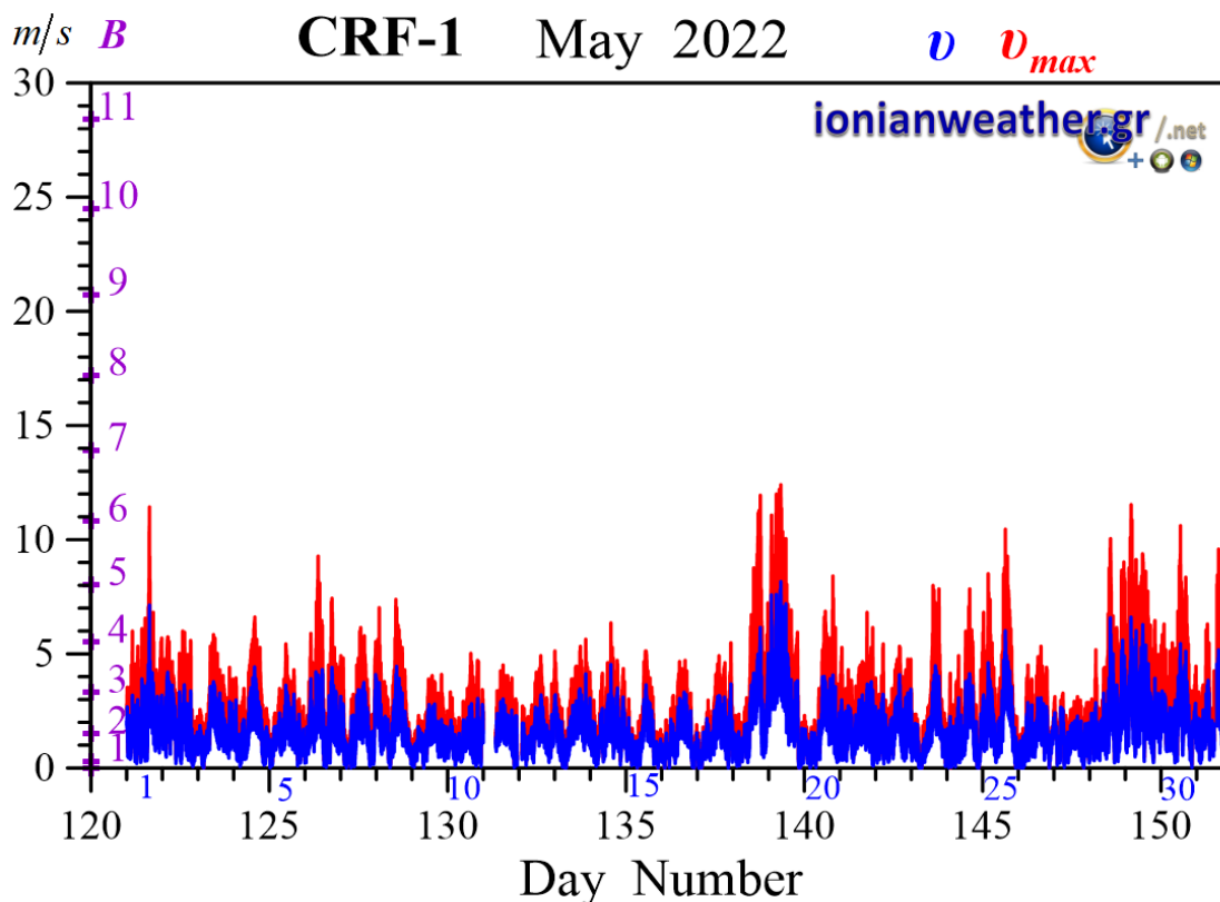
Εικόνα CRF1-2: Μέση ανά λεπτό ταχύτητα ανέμου ( m/s , γαλάζιο) και ριπή ανέμου (κόκκινο) Μαΐου 2022. Κλίμακα ταχυτήτων αριστερά σε m/s και Beaufort .
