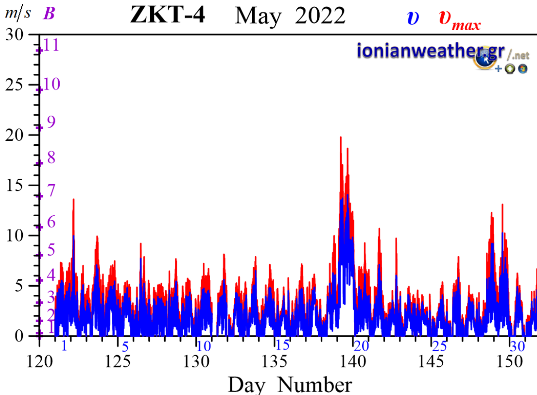
Εικόνα ZKT4-2: Μέση ανά λεπτό ταχύτητα ανέμου (m/s, γαλάζιο) και ριπή ανέμου (κόκκινο) Μαΐου 2022. Κλίμακα ταχυτήτων αριστερά σε m/s και Beaufort.
