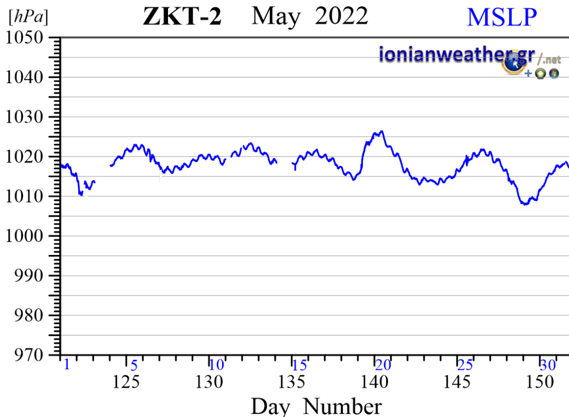
Εικόνα ZKT2-6: Μέση ανά λεπτό βαρομετρική πίεση Μαΐου 2022 ανηγμένη στην επιφάνεια της θάλασσας.
