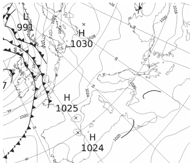
Εικόνα 3.1-10: MSLP 10 May 2022 00UTC
