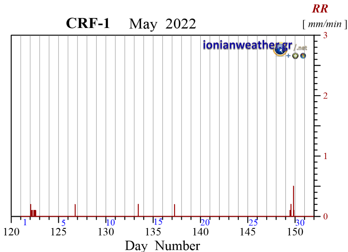
Εικόνα CRF1-1: Ανά λεπτό ρυθμός βροχόπτωσης ( mm/min ) Μαΐου 2022.
