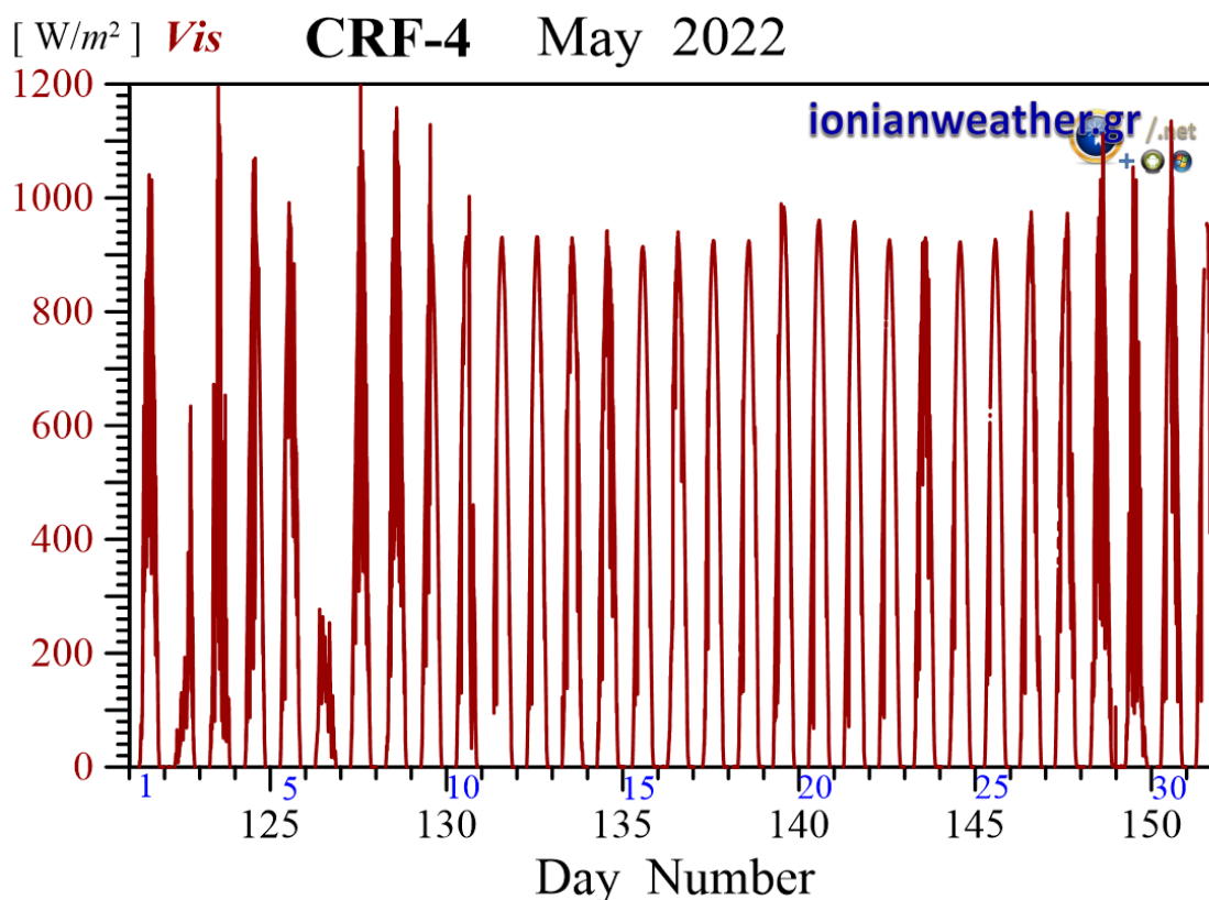
Εικόνα CRF4-7: Μέση ανά λεπτό Ηλιακή ακτινοβολία Μαΐου 2022 στην οπτική και εγγύς υπέρυθρη περιοχή.
