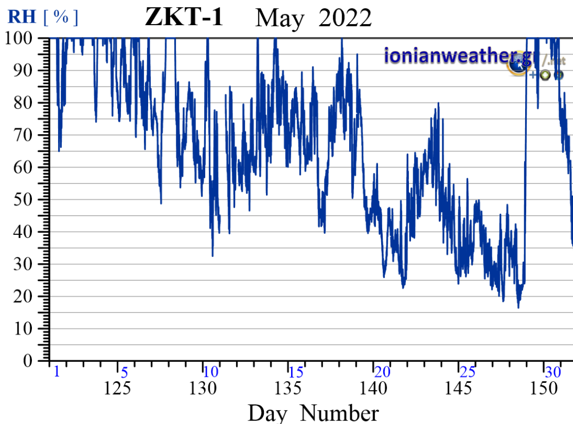
Εικόνα ZKT1-5: Μέση ανά λεπτό σχετική υγρασία Μαΐου 2022.
