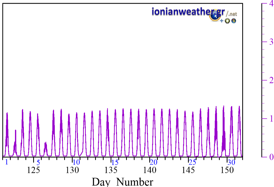
Εικόνα CRF1-9: Μέση ανά λεπτό Ηλιακή ακτινοβολία Μαΐου 2022 στη φασματική περιοχή UVB.
