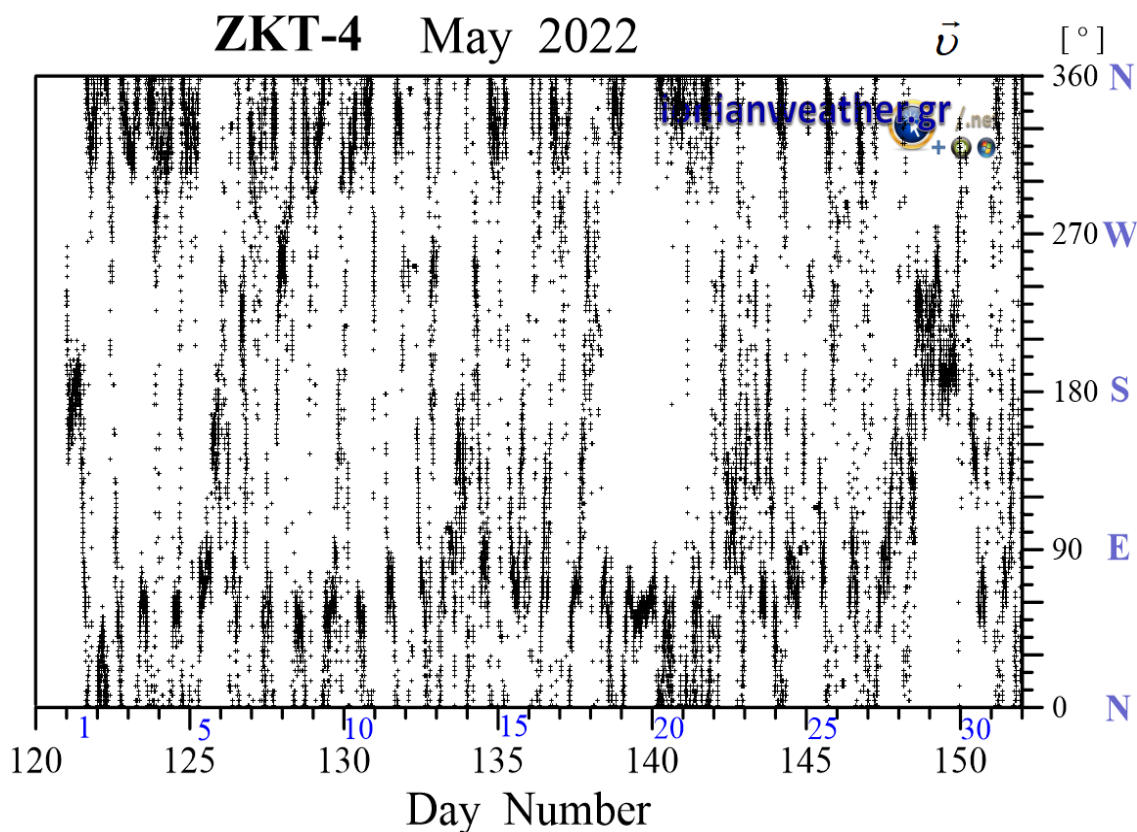
Εικόνα ZKT4-3: Μέση ανά λεπτό κατεύθυνση ανέμου Μαΐου 2022 (κλίμακα αζιμουθίων δεξιά)
