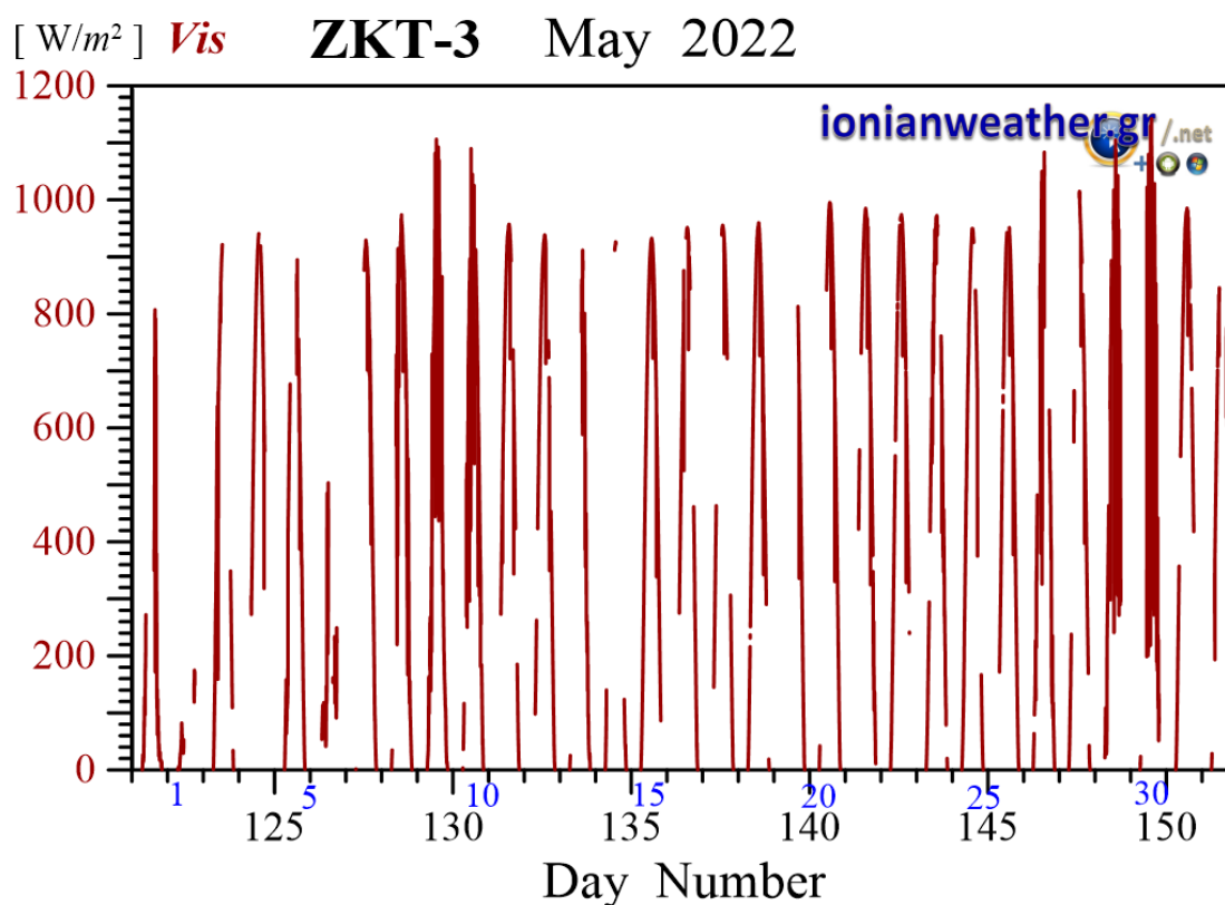
Εικόνα ZKT3-7: Μέση ανά λεπτό Ηλιακή ακτινοβολία Μαΐου 2022 στην οπτική και εγγύς υπέρυθρη περιοχή.
