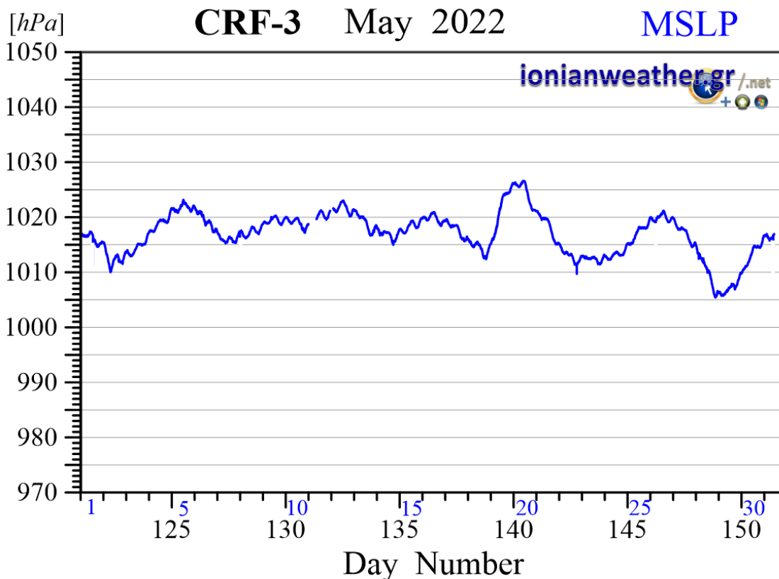
Εικόνα CRF3-6: Μέση ανά λεπτό βαρομετρική πίεση Μαΐου 2022 ανηγμένη στην επιφάνεια της θάλασσας.
