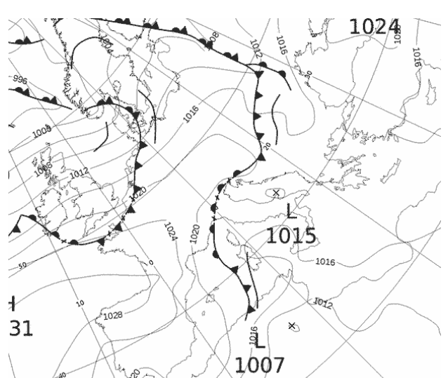
Εικόνα 3.1-26: MSLP 26 May 2022 00UTC
