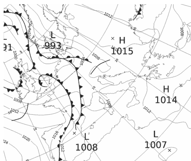
Εικόνα 3.1-24: MSLP 24 May 2022 00UTC
