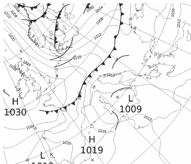
Εικόνα 3.1-28: MSLP 28 May 2022 00UTC
