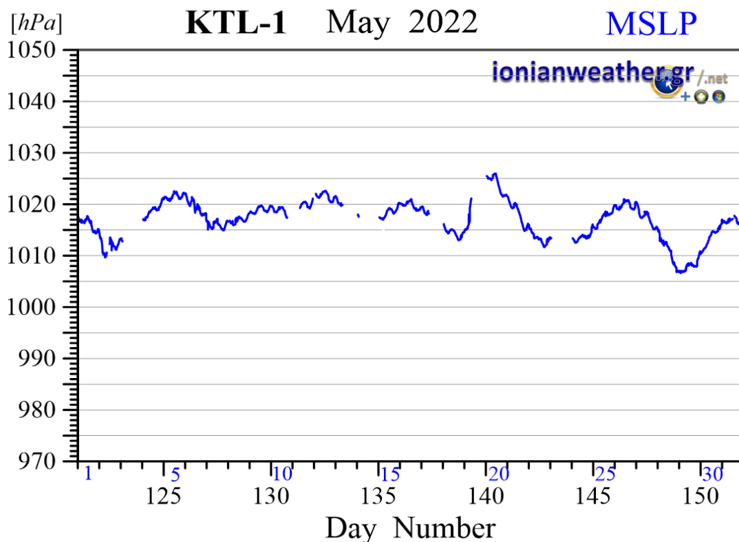
Εικόνα KTL1-6: Μέση ανά λεπτό βαρομετρική πίεση Μαΐου 2022 ανηγμένη στην επιφάνεια της θάλασσας.
