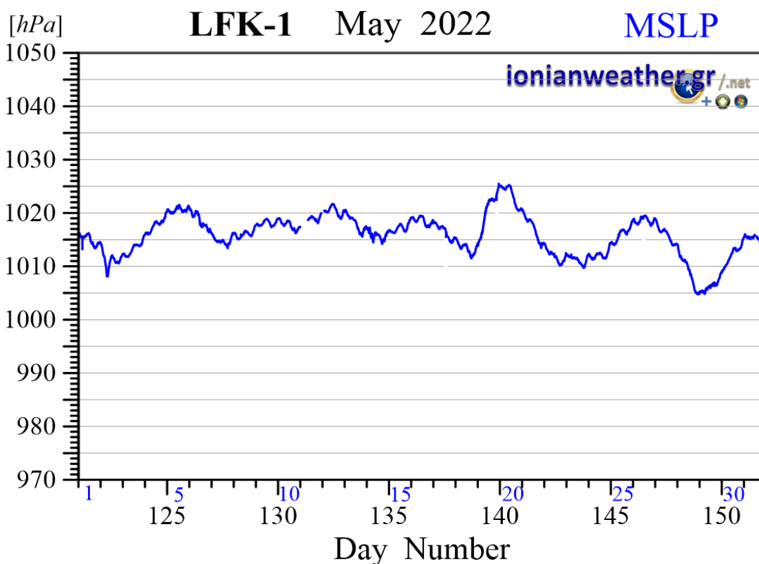
Εικόνα LFK1-6: Μέση ανά λεπτό βαρομετρική πίεση Μαΐου 2022 ανηγμένη στην επιφάνεια της θάλασσας.
