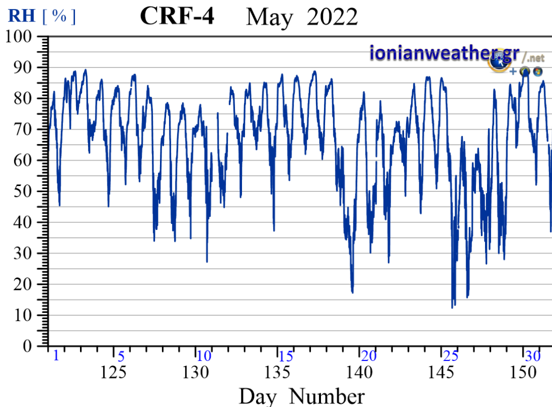
Εικόνα CRF4-5: Μέση ανά λεπτό σχετική υγρασία Μαΐου 2022.
