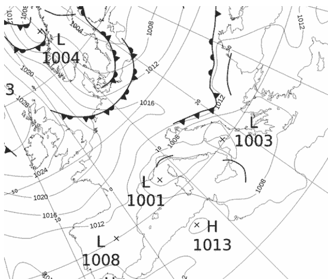
Εικόνα 3.1-29: MSLP 29 May 2022 00UTC
