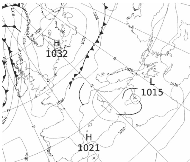
Εικόνα 3.1-9: MSLP 9 May 2022 00UTC
