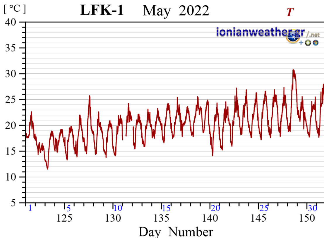
Εικόνα LFK1-4: Μέση ανά λεπτό θερμοκρασία αέρα Μαΐου 2022.
