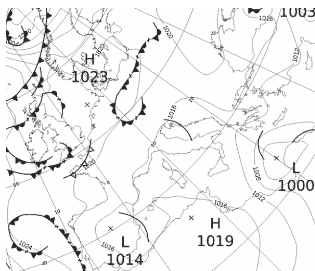
Εικόνα 3.1-2: MSLP 2 May 2022 00UTC
