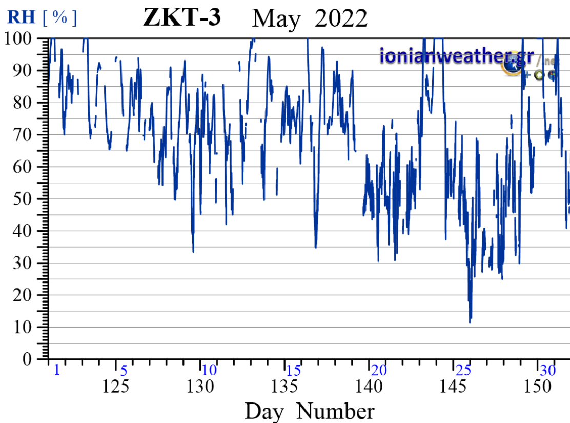
Εικόνα ZKT3-5: Μέση ανά λεπτό σχετική υγρασία Μαΐου 2022.
