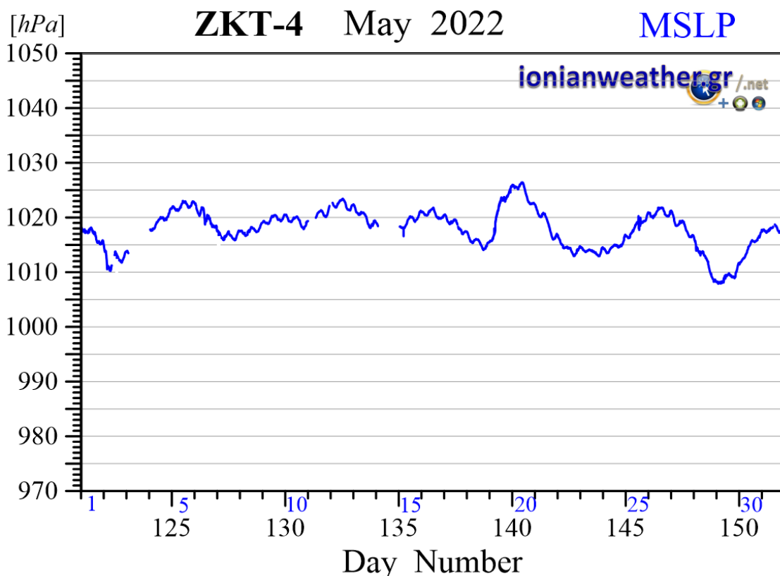
Εικόνα ZKT4-6: Μέση ανά λεπτό βαρομετρική πίεση Μαΐου 2022 ανηγμένη στην επιφάνεια της θάλασσας.
