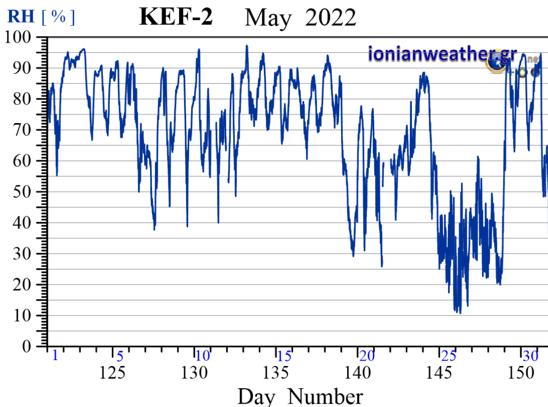
Εικόνα KEF2-5: Μέση ανά λεπτό σχετική υγρασία Μαΐου 2022.
