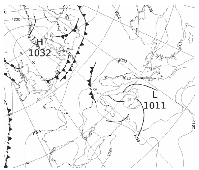
Εικόνα 3.1-8: MSLP 8 May 2022 00UTC
