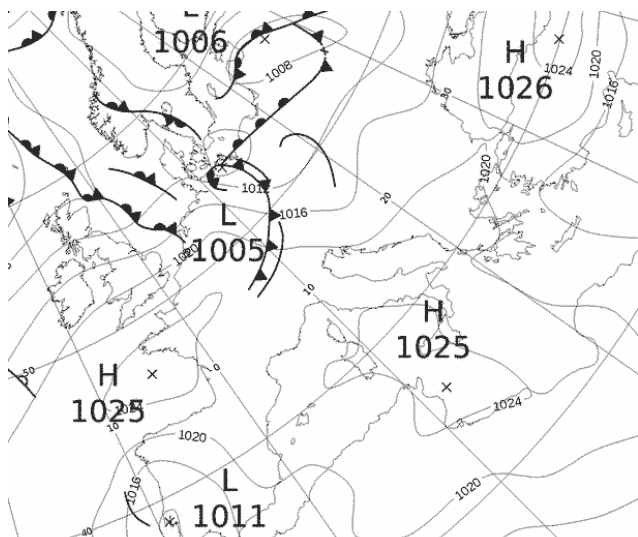
Εικόνα 3.1-21: MSLP 21 May 2022 00UTC
