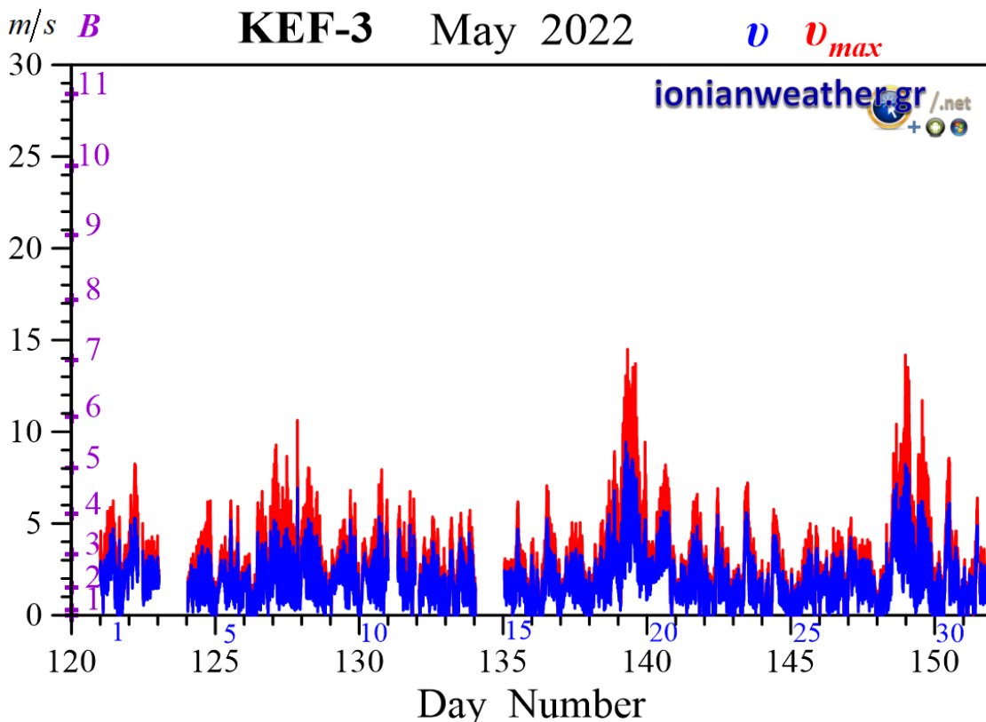
Εικόνα KEF3-2: Μέση ανά λεπτό ταχύτητα ανέμου (m/s, γαλάζιο) και ριπή ανέμου (κόκκινο) Μαΐου 2022. Κλίμακα ταχυτήτων αριστερά σε m/s και Beaufort.
