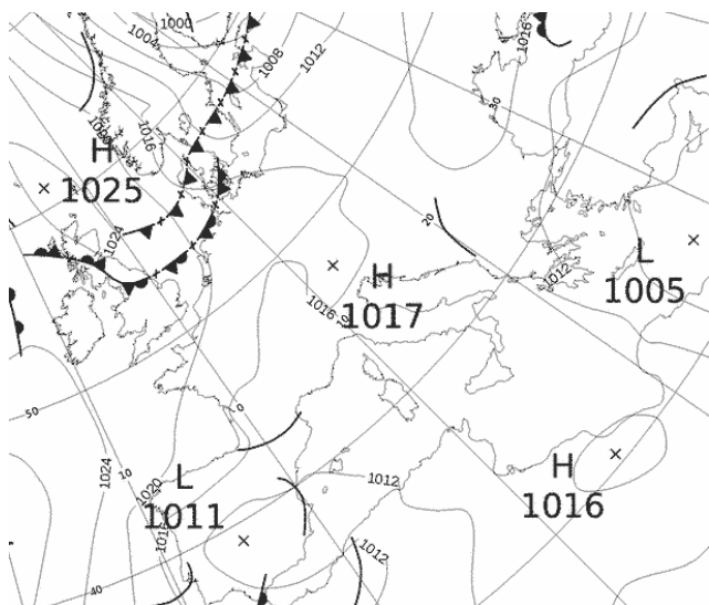
Εικόνα 3.1-3: MSLP 3 May 2022 00UTC
